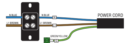
220-240V 2 CABLES + TIERRA
