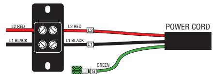
240V 2 CABLES + TIERRA
