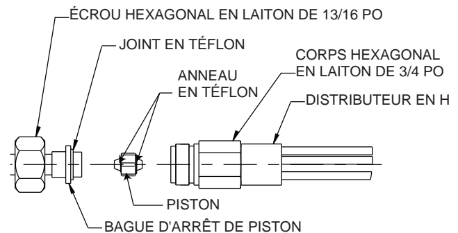
Figure 5 – Piston intérieur (climatisation)
