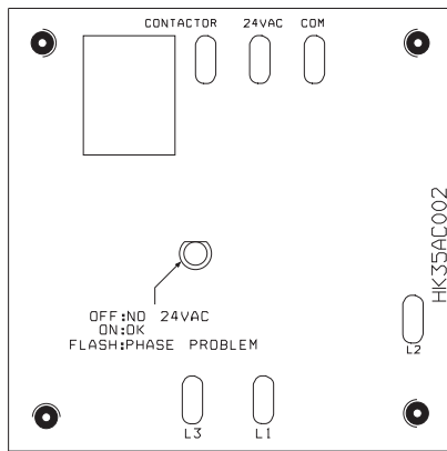
Figure 7 – Commande de moniteur triphasé (s'applique aux appareils triphasés seulement)
