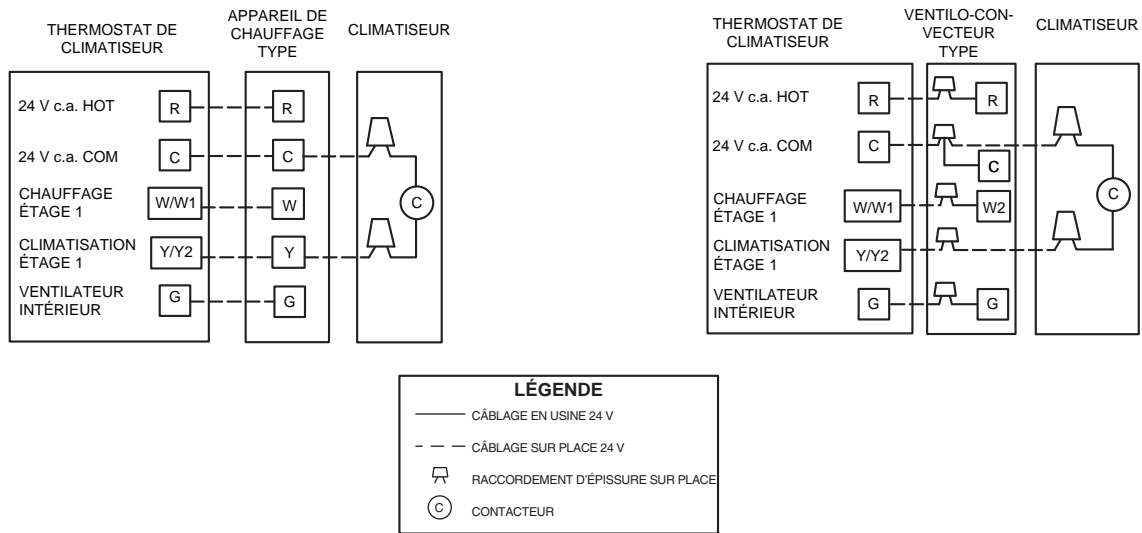
Fig. 8 – Schémas de câblage génériques (consultez les instructions d'installation du thermostat pour connaître les combinaisons spécifiques des appareils)
