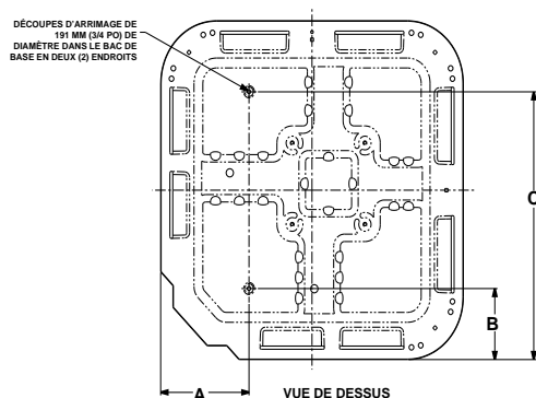
Fig. 2 – Emplacements des découpes d'arrimage
