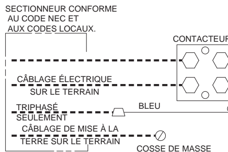
Fig. 6 – Raccords de conduite
