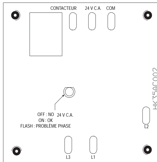
Fig. 7 – Panneau de moniteur pour appareils triphasés (uniquement pour les appareils triphasés)
