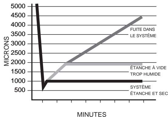
Fig. 4 – Courbe de vide
