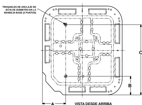
Fig. 2 – Ubicaciones de los troqueles de anclaje
