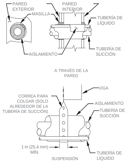
Fig. 1 – Instalación de tuberías
