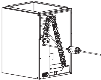
Fig. 3 – Filtro secador de la tubería de líquidos
