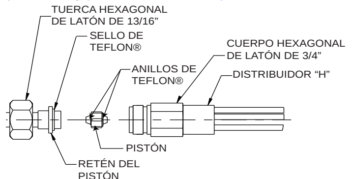
Fig. 5 – Fig. 5: Pistón para interiores (enfriamiento)
