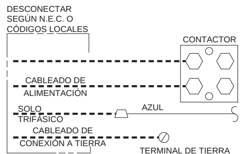
Fig. 6 – Fig. 6: Conexiones de la línea Conexión del cableado de control
