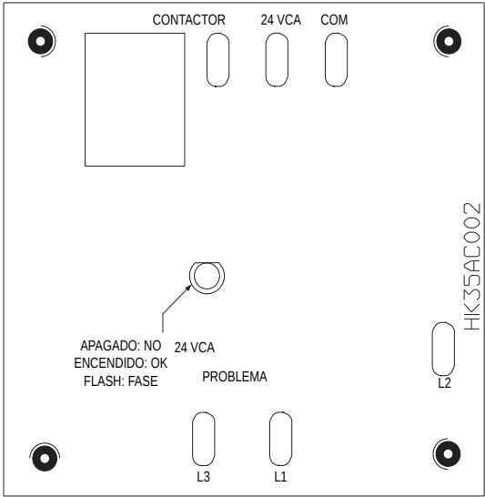
Fig. 7 – Control de monitor trifásico (Se aplica solo a unidades trifásicas)
