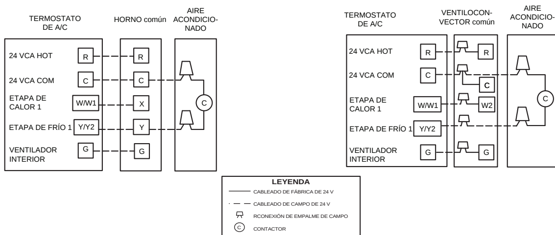
Fig. 8 – Diagramas de cableado genéricos (Consulte las instrucciones de instalación del termostato para conocer las combinaciones de unidades específicas)
