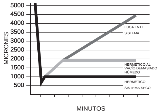
Fig. 4 – Fig. 4: Gráfico de vacío profundo
