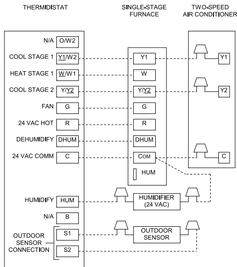
Figure 6 – Câblage du thermostat avec climatiseur à 2 étages et frigorigène Puron
