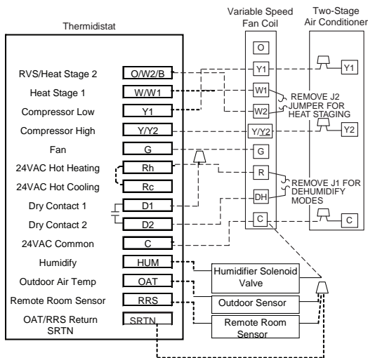
Thermostat Edge modèles TP-PRH-01 et TP-NRH-01 avec ventilateur-convecteur et climatiseur 2 étages
