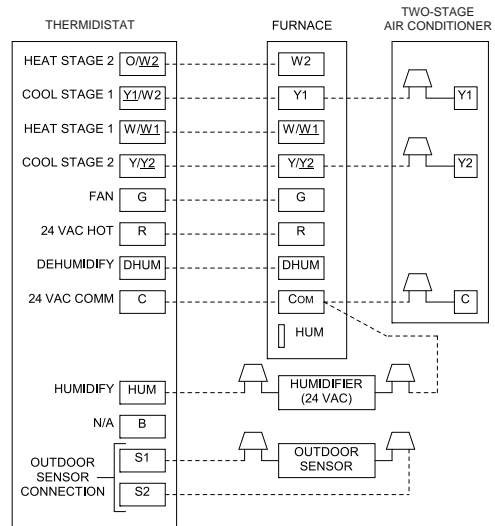
Thermostat modèle TSTATCCPRH01-B avec appareil de chauffage VS et climatiseur 2 étages
