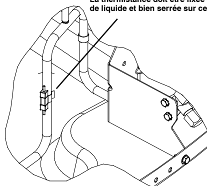
Fig. 10 – Accessoire de thermistance de serpentin extérieur (OCT)
