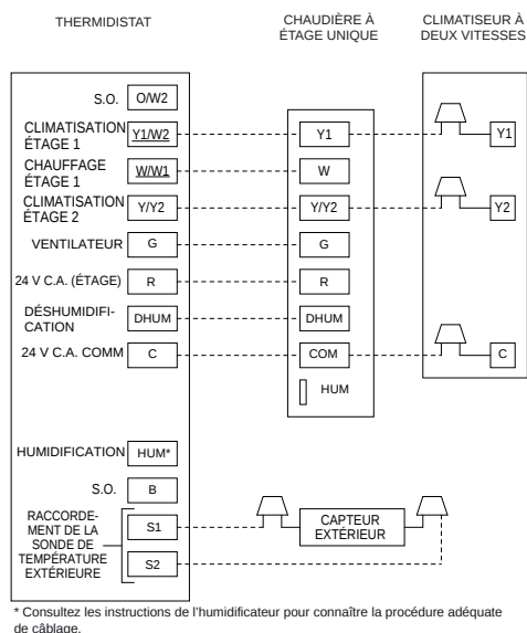
Fig. 11 – Câblage du thermostat avec climatiseur 2 étages et frigorigène Puron (configuré en tant que système non communicant)
