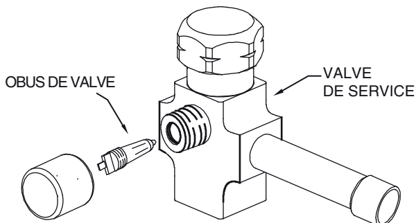
Figure 5 – Valve de service de vapeur
