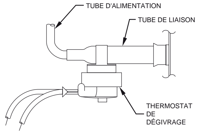
Fig. 3 – Emplacement du thermostat de dégivrage
