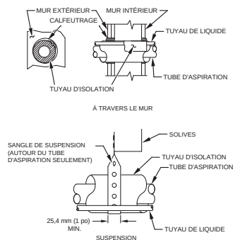
Figure 1 – Installation des conduites
