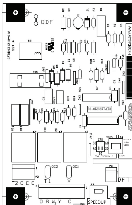
Figure 12 – Commande de dégivrage HK32EA010
