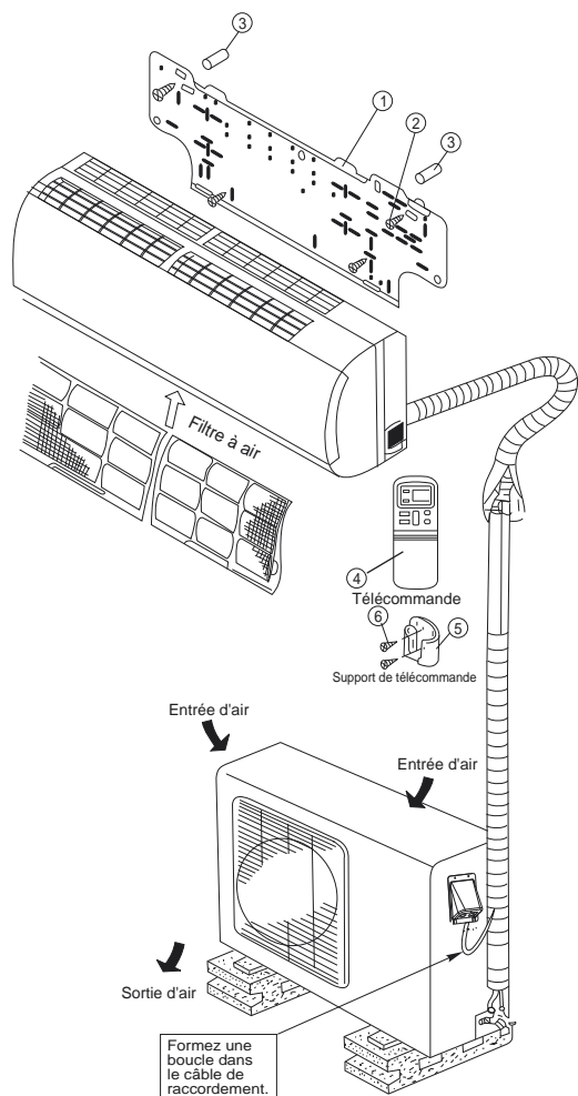
Fig. 1 – 40MVC, MVQ/38MVC et MVQ009-012 Liste de pièces
