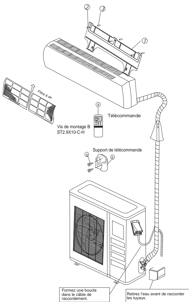
Fig. 2 – 40MVC, MVQ/38MVC et MVQ018-024 Liste de pièces
