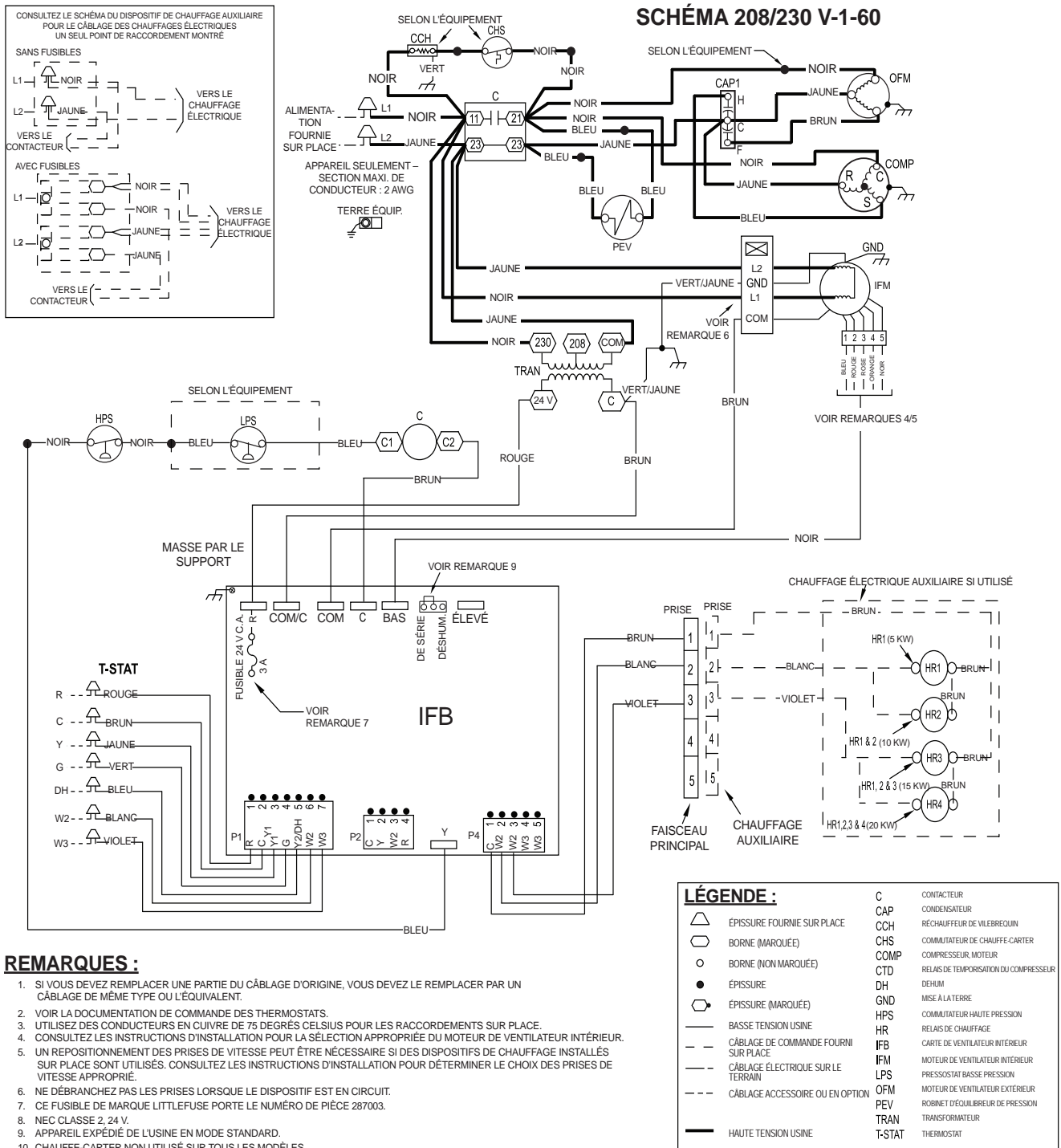
Figure 14 – Schéma de connexion de câblage – 208/230-1-60 – Capacités -30
