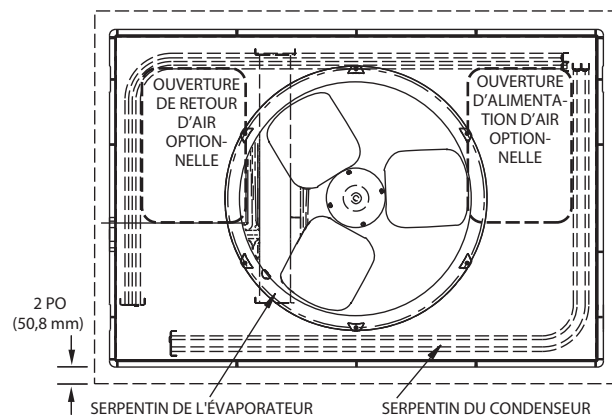
Figure 7 – Détails du montage sur dalle
