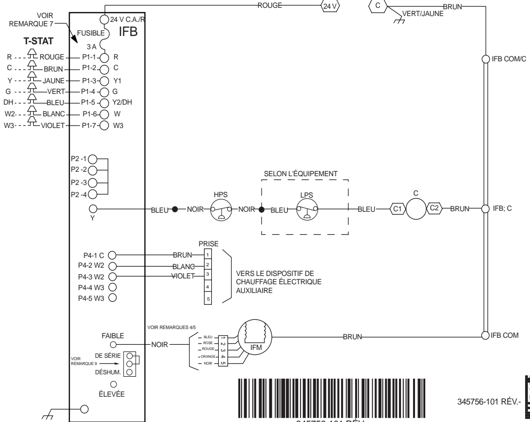
Figure 15 – Schéma de câblage en échelle – 208/230-1-60 – Capacités -30
