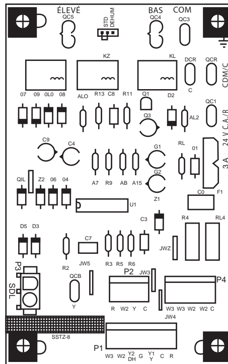
Figure 11 – Carte interface du ventilateur (IFB) Refroidissement à vitesse unique avec vitesse supérieure en mode de chauffage électrique
