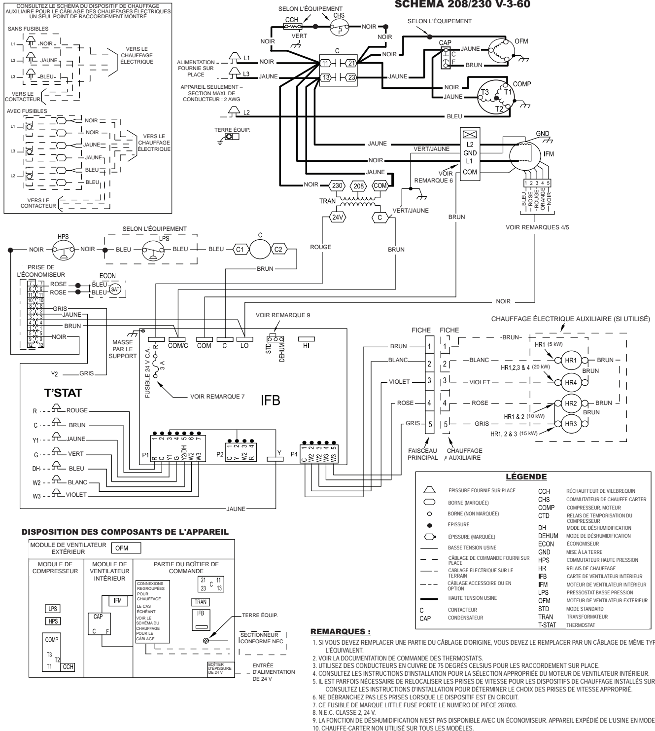
Figure 16 – Schéma de connexion de câblage – 208/230-3-60
