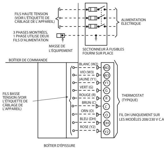
Figure 10 – Branchements haute et basse tensions
