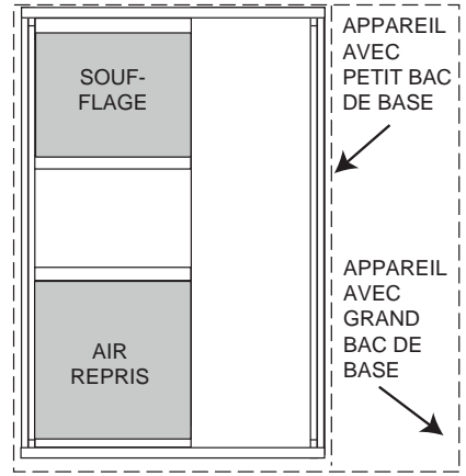
POSE DE L'APPAREIL SUR UN CADRE COMMUN
