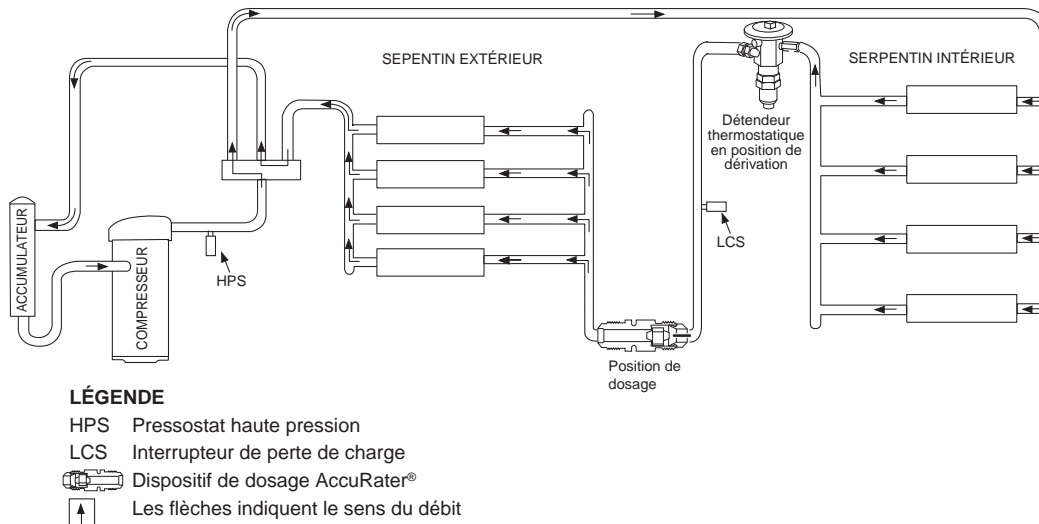
Figure 13 – Fonctionnement typique de la thermopompe, mode de chauffage
