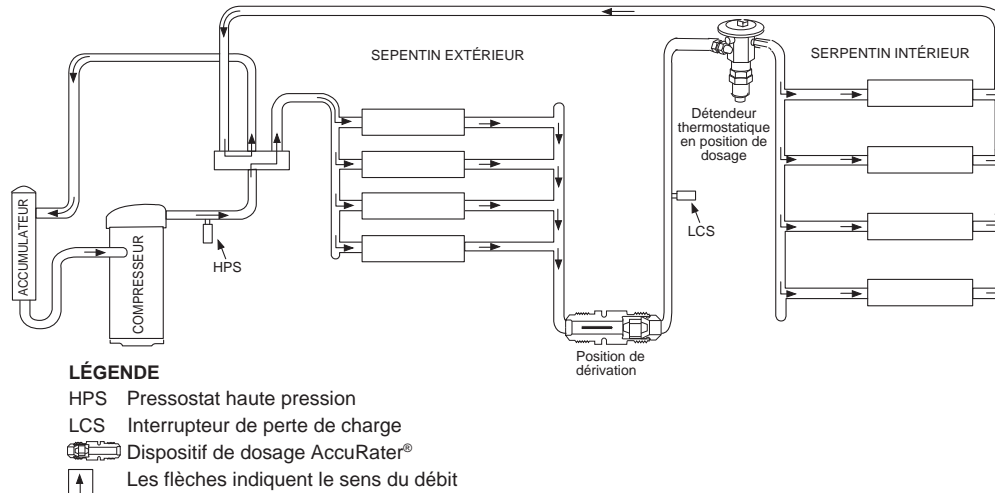
Figure 14 – Fonctionnement typique de la thermopompe, mode de refroidissement
