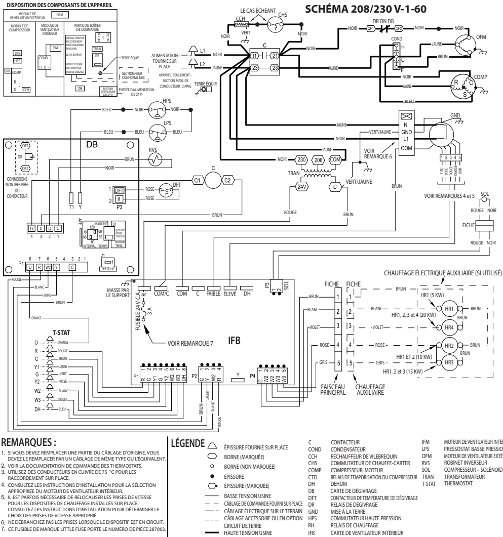
Figure 15 – Schéma de connexion de câblage sans FIOP de déshumidification avancée - 208/230-1-60
