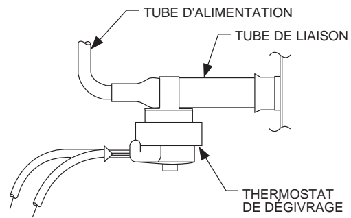
Figure 22 – Thermostat de dégivrage
