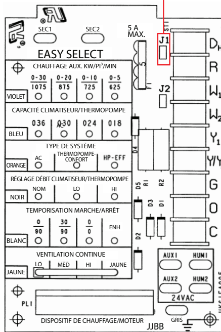
Figure 11 – Carte interface du ventilateur (IFB)
