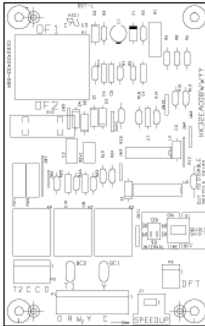
Figure 12 – Carte de dégivrage
