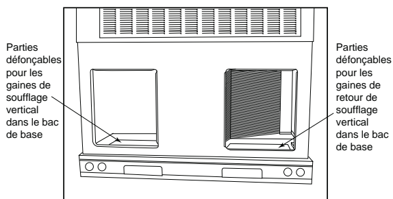
Figure 9 – Ouvertures d'air de soufflage et de retour
