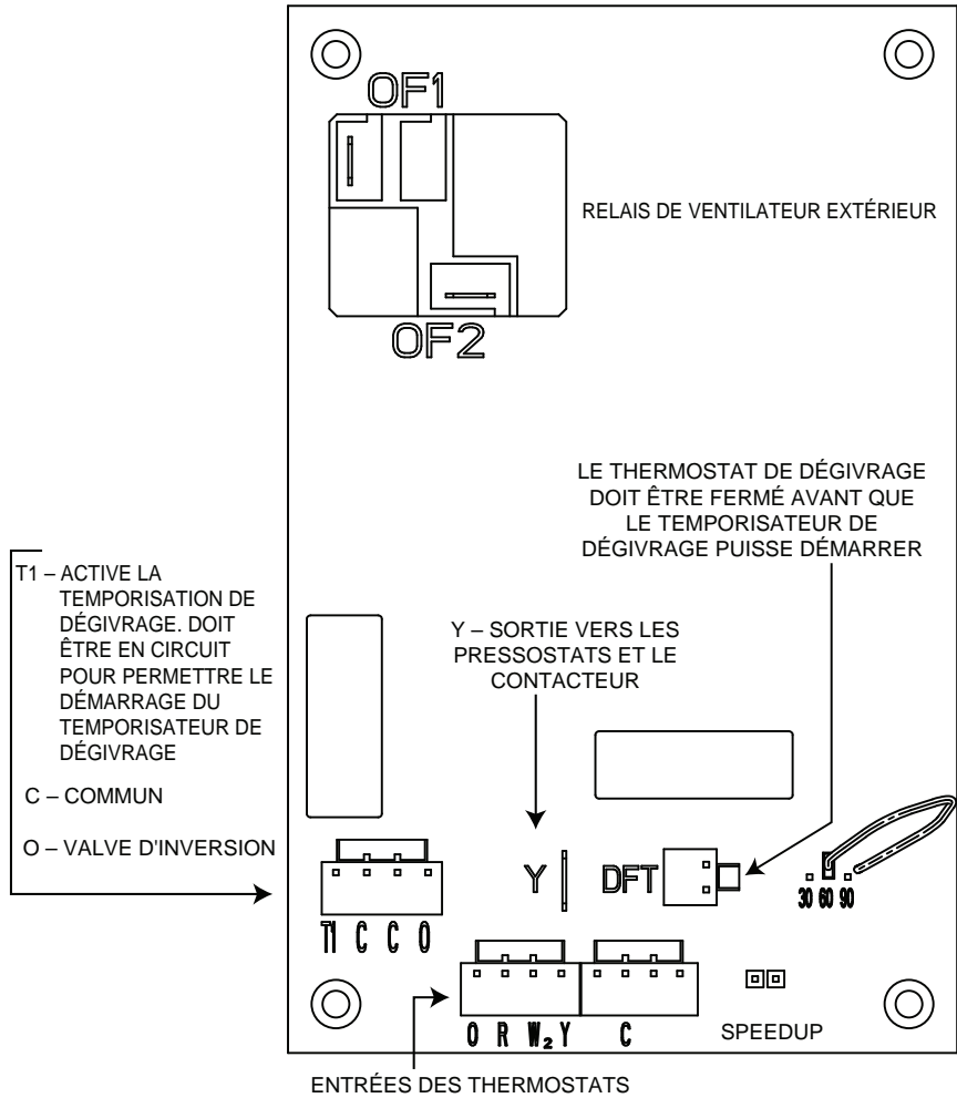
Figure 19 - Commande de dégivrage
