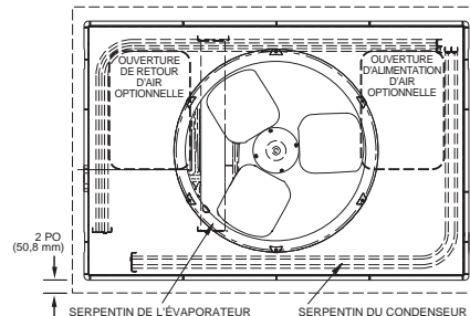
Figure 8 – Détails du montage sur dalle
