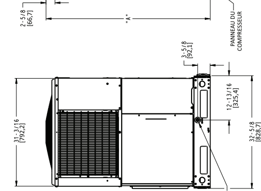
VUE DU CÔTÉ GAUCHE
