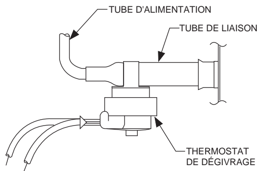
Figure 23 – Thermostat de dégivrage
