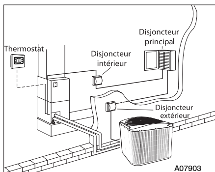
Fig. 1 - Disjoncteurs
