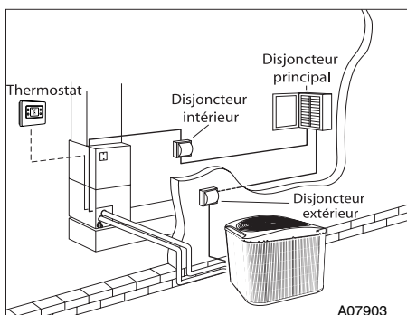
Fig. 1 - Disjoncteurs
