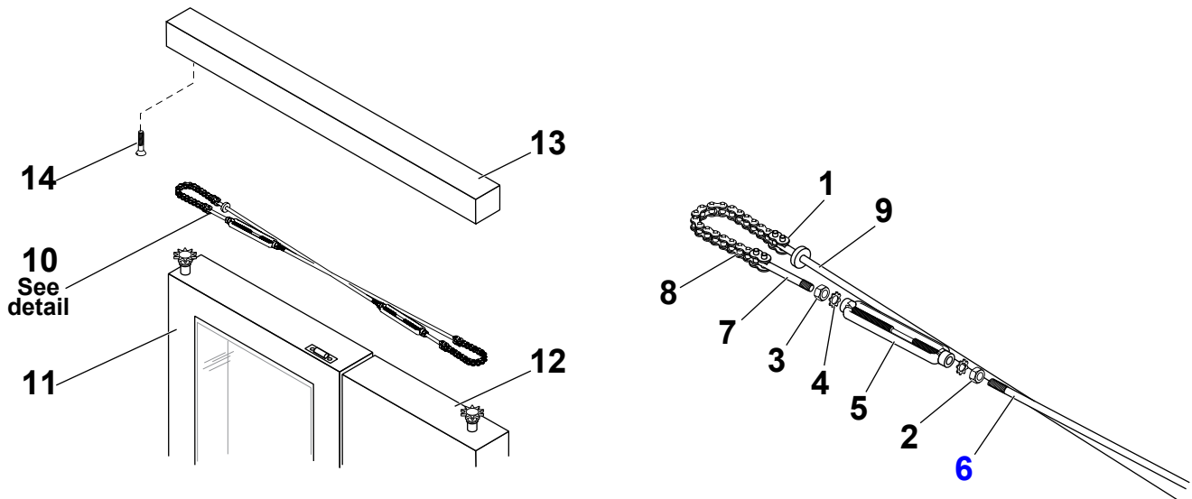
Figure: PL-2 Door Assembly (65/35 Door Units)
