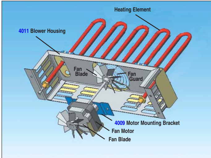
BLD FAN AL 3" Fan Blade
