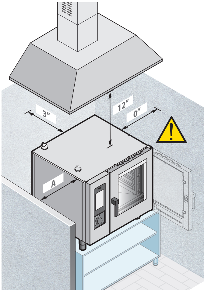
A - 20" installazione- manutenzione / 3" uso A - 20" installation - maintenance / 3" use
