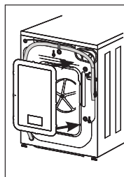
Replacer la plaque arrière et ses 4 vis de fixation
