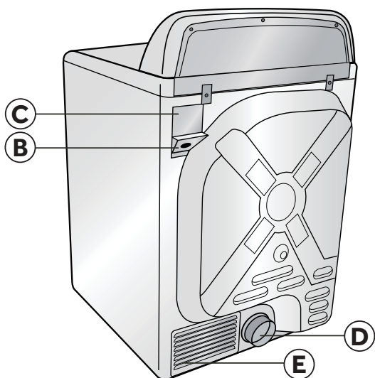
Secadora eléctrica
