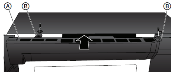
(A) Mazo de alambres (no se muestra) (B) Lengüeta del orificio de los tornillos (2)
