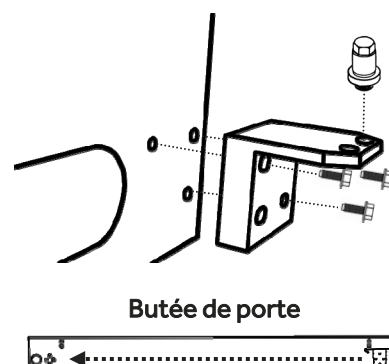
Charnière inférieure
