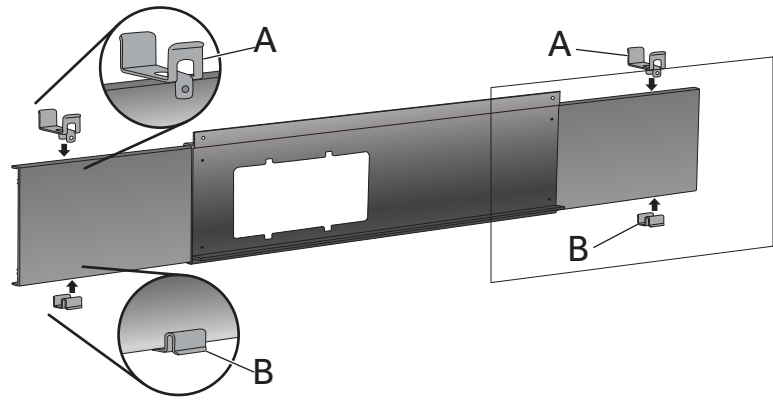
(A) Soportes superiores de la ventana
