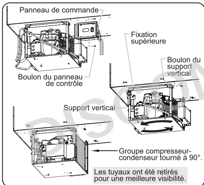
Rotation du groupe compresseur-condenseur
