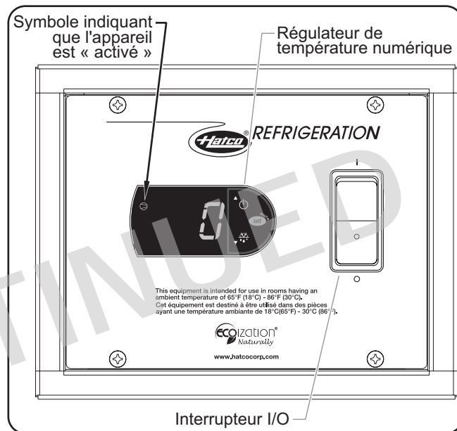
Panneau de contrôle des séries CWB
