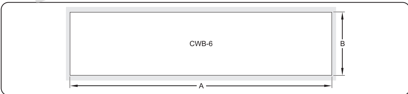
Dimensions de découpe du comptoir pour séries CWB
