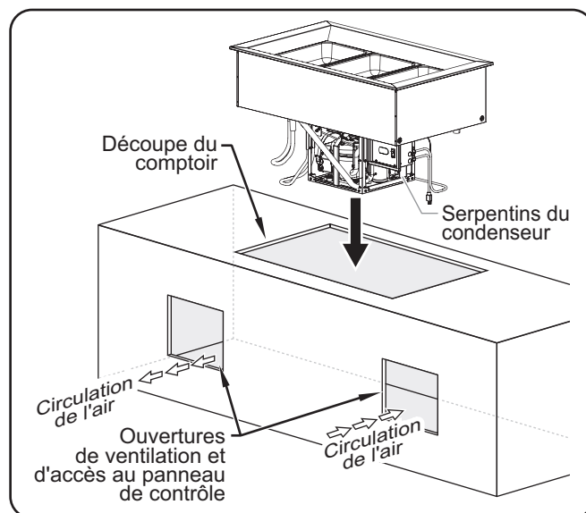
Installation d'un modèle CWB-3
