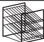
Présentoir Incliné à 3 Niveaux Ouvertures de présentoir : 89 mm (3-1/2") Le niveau central est amovible. Les niveaux sont inclinés à 15°.
