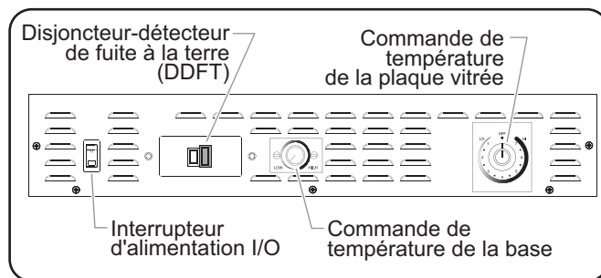
Commandes pour GRHW-1SGD et GRHW-1SGDS (commandes GRHW-1SGS illustrées)
