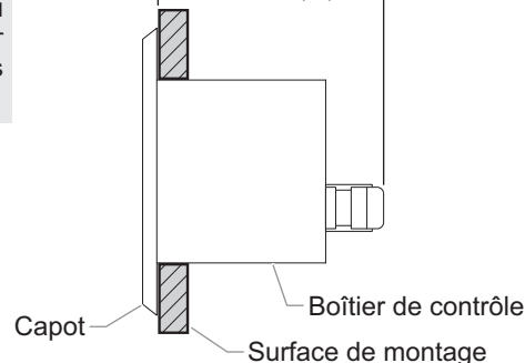
Vue de côté du boîtier installé
