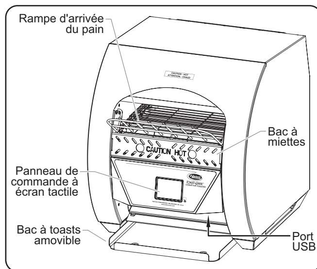
Grille-pain à convoyeur modèle TQ3-400
