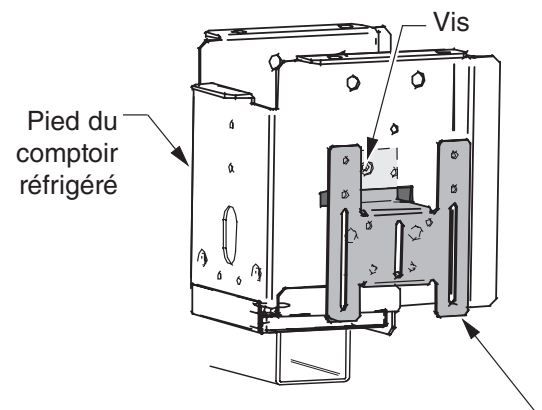
Support de la plinthe d'extrémité (le rebord s'accroche dans la fente du pied du comptoir réfrigéré)
