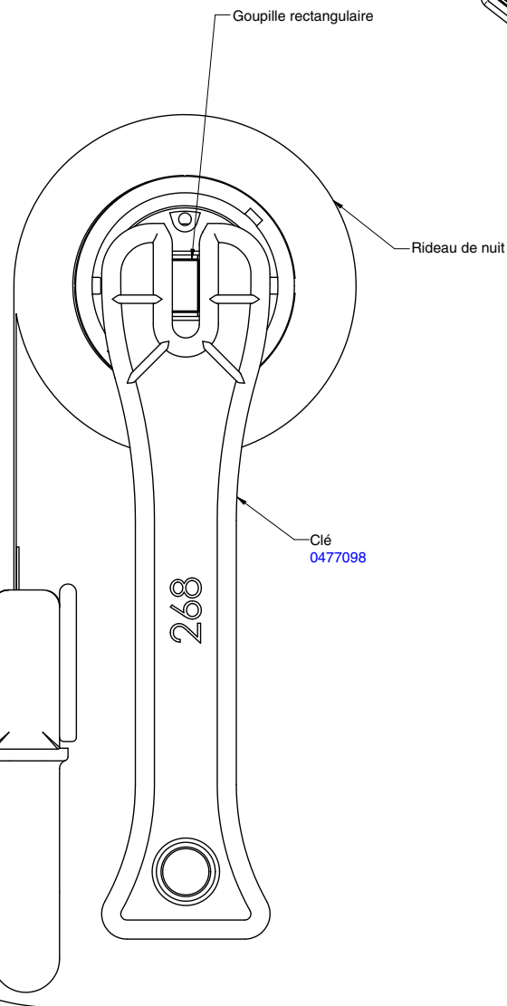
Goupille rectangulaire
