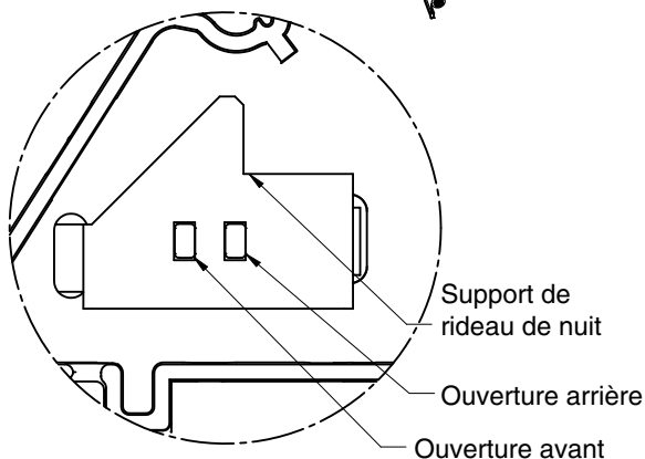
Détail A
