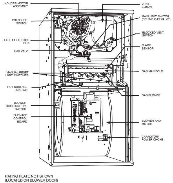
Fig. 1 – 80% AFUE Single Stage Furnace Components
