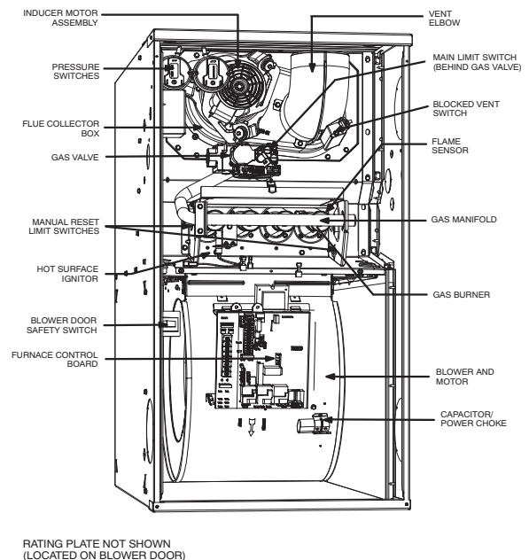
Fig. 2 – 80% AFUE Two-Stage Furnace Components
