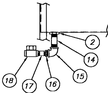
VIEW A-A
