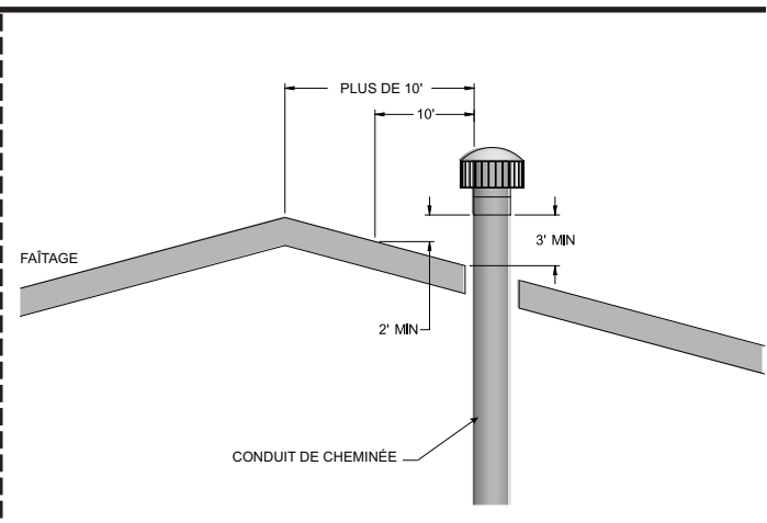
Figure 2-2 Terminaison de ventilation depuis un toit à double pente - 10 pi. ou plus du faîtage
