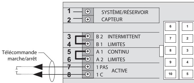
Figure 5-7_Chaudière à deux étages (puissance maxi/mini)
