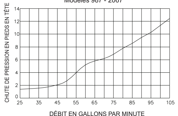
DIAGRAMME DE CHUTE DE PRESSION Modèles 987 - 2067
