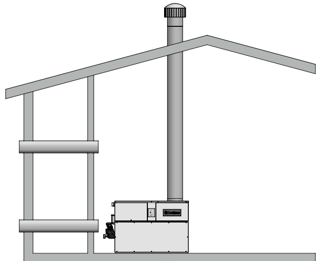
Figure 1-7 _Air de combustion extérieur, avec conduites
