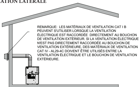
VENTILATION LATÉRALE
