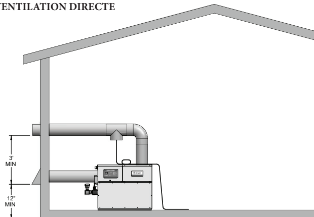
VENTILATION DIRECTE
