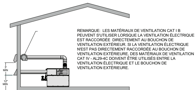
VENTILATION HORIZONTALE D'AIR DIRECT
