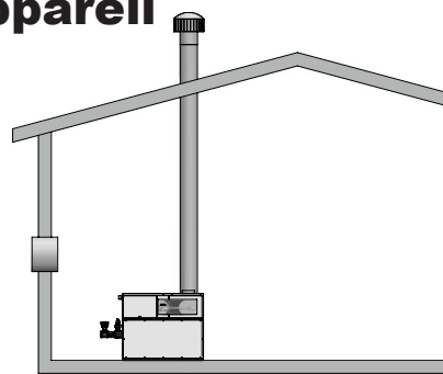
Figure 1-2_Air extérieur de combustion - Ouverture unique Deux ouvertures
