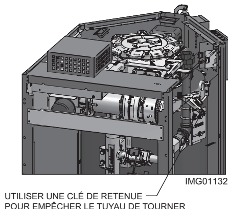
Figure 6-2 Tuyau d'entrée avec clé de retenue
