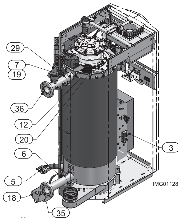
Vue arrière
