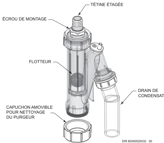
Figure 2-1 Purgeur de condensat
