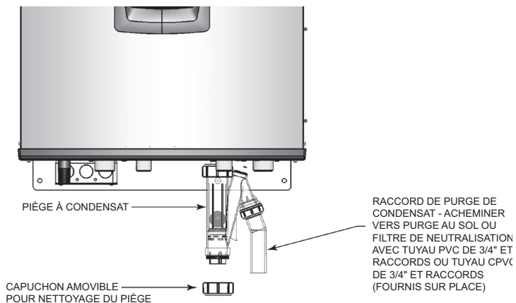
Figure 2-2 Élimination du condensat
