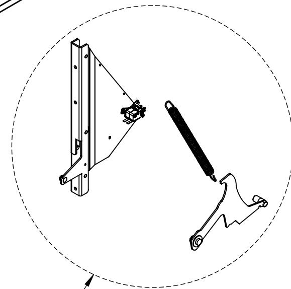
DOOR HINGE ASSEMBLY RHS
