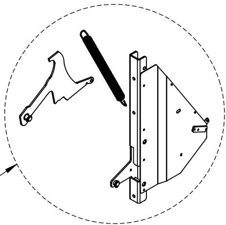
DOOR HINGE ASSEMBLY LHS
