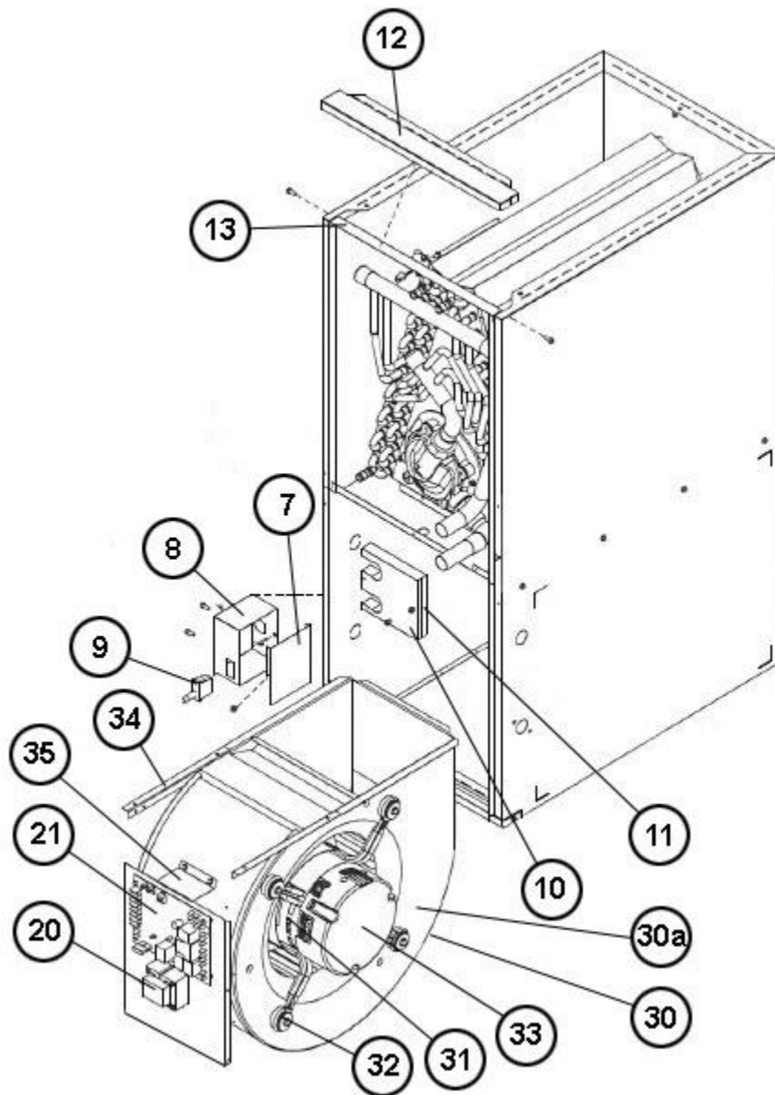
Cabinet-Blower Assembly
