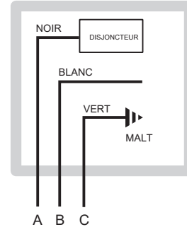
Figure 25. Raccordements d'alimentation
