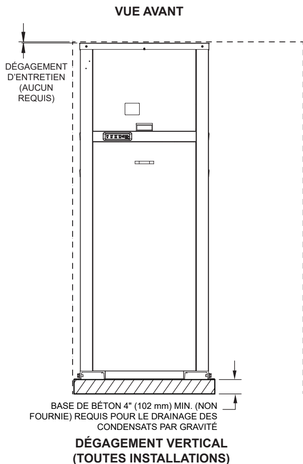
Figure 6. Dégagements minimum aux matières combustibles – Installation intérieure ou extérieure
