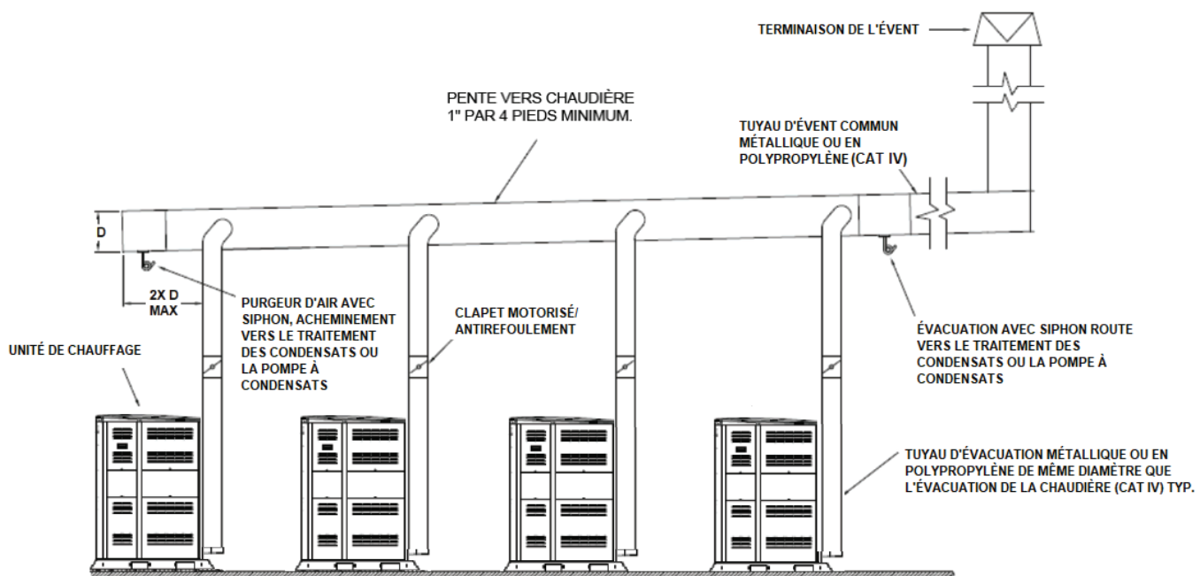
Figure 74. Événement commun à pression positive typique
