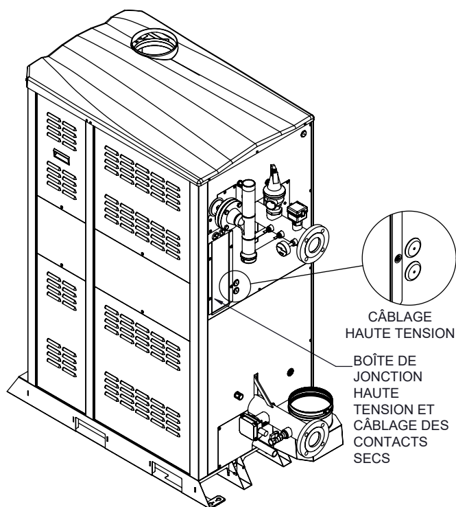
Figure 37. Emplacement boîte de jonction arrière
