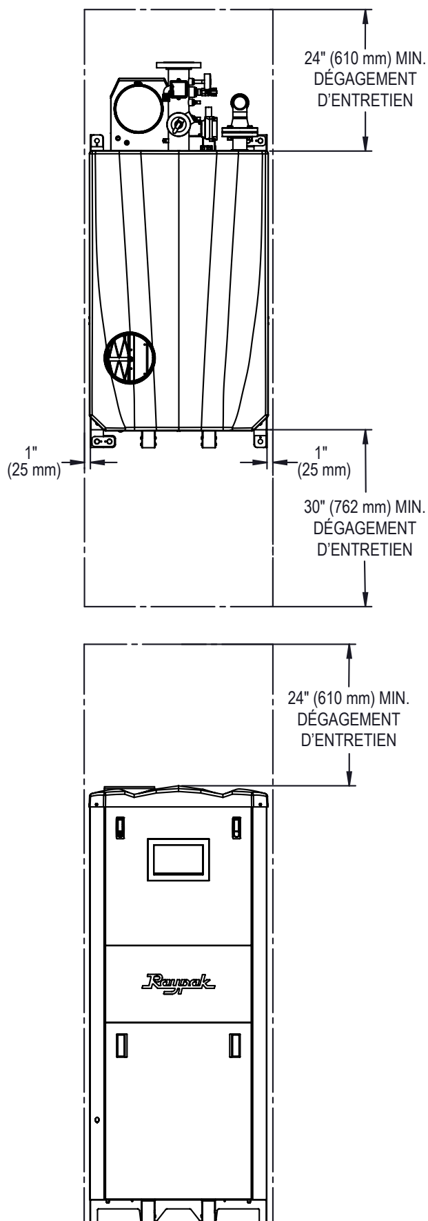
Figure 8. Dégagements minimum aux matières combustibles – Installation intérieure ou extérieure
