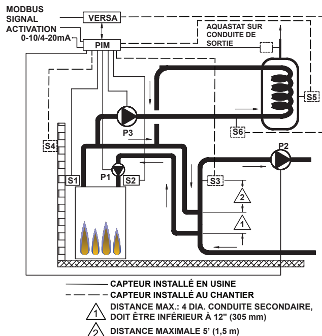
Figure 29. Mode 3 - Chaudière unique avec chauffe-eau indirect sur boucle primaire - boucles prim./sec.
