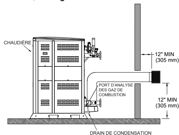
Figure 65. Acier inoxydable et polypropylène - Ventilation directe murale à l'horizontale
