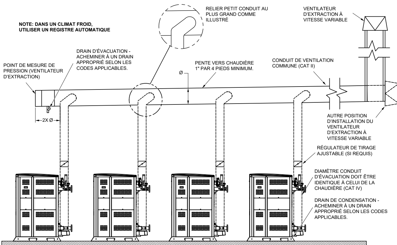
Figure 73. Évent commun à pression négative typique
