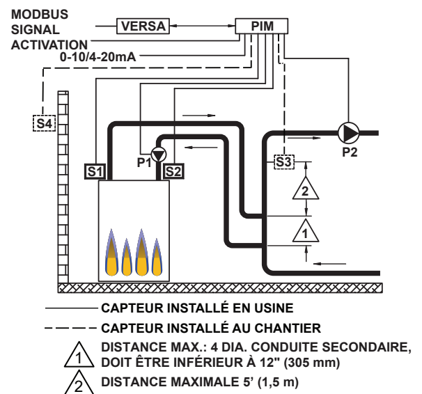
Figure 26. Mode 1 - Chaudière unique avec boucles primaire/secondaire
