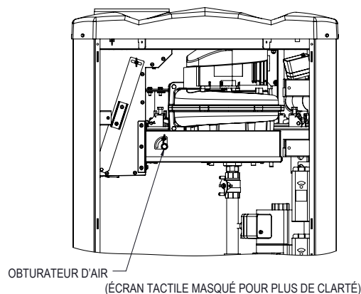
Figure 106. Réglage de l'obturateur d'air
