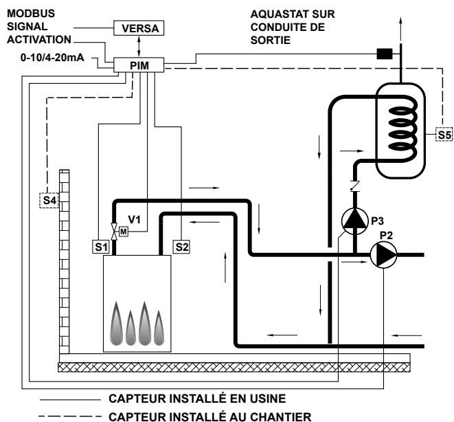
Figure 35. Mode 2 - Chaudière unique avec chauffe-eau indirect - boucle primaire
