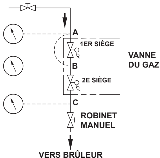
Figure 107. Essai d'étanchéité
