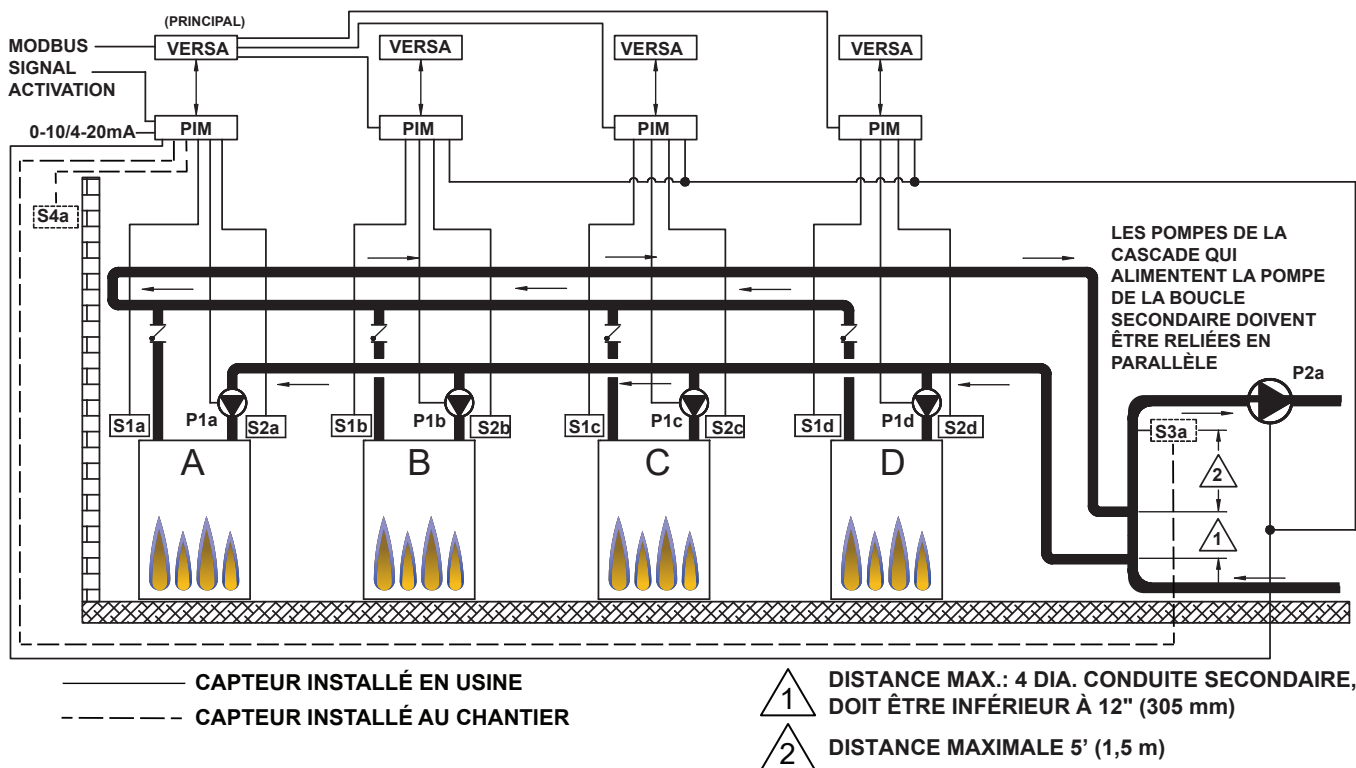
Figure 27. Mode 1 - Cascade de chaudières recommandée (jusqu'à 8 appareils) - boucles prim./sec.
