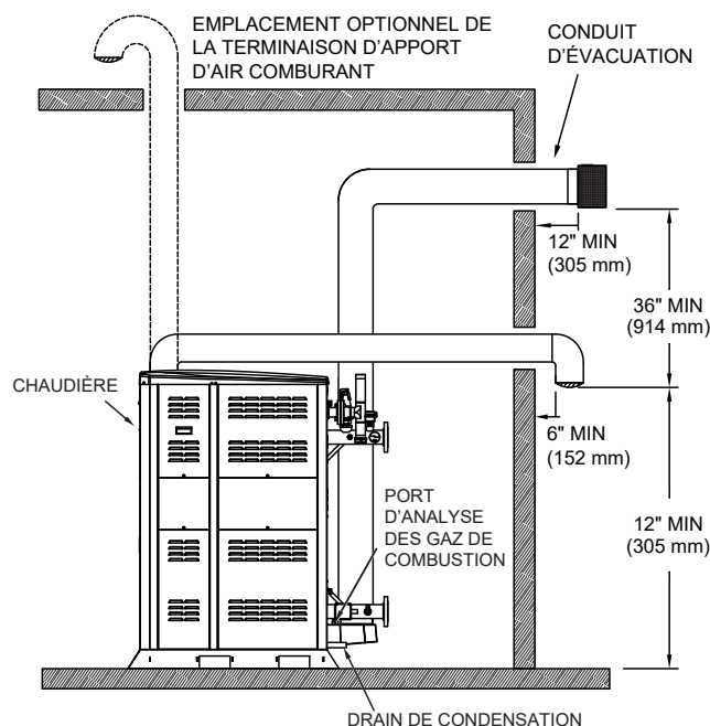
Figure 66. Acier inoxydable et polypropylène - Ventilation directe à l'horizontale
