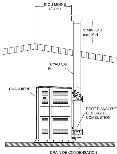
Figure 63. Acier inoxydable et polypropylène - Ventilation verticale
