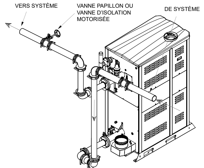
Figure 30. Tuyauterie primaire hydronique
