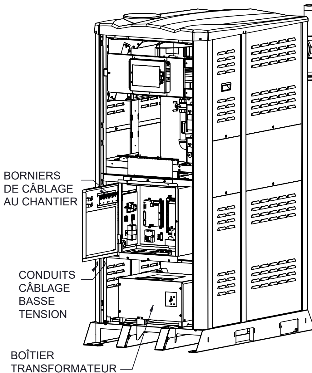
Figure 50. Boîtier de jonction basse tension
