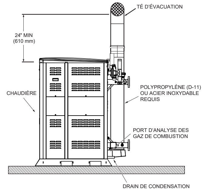
Figure 72. Installation extérieure (kit d'évacuation extérieure Polypro D-11)
