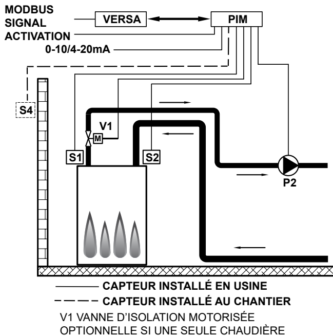
Figure 31. Mode 1 - Chaudière unique avec boucle primaire
