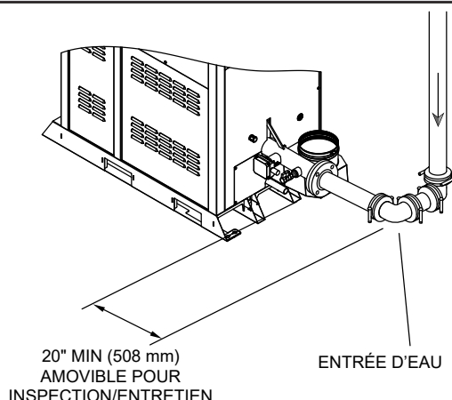
Figure 19. Exigence de tuyauterie
