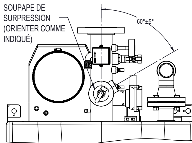
Figure 22. Orientation recommandée de la soupape
