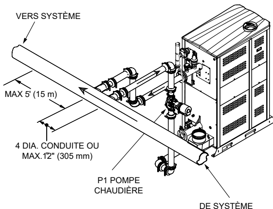
Figure 25. Boucles primaire/secondaire hydroniques
