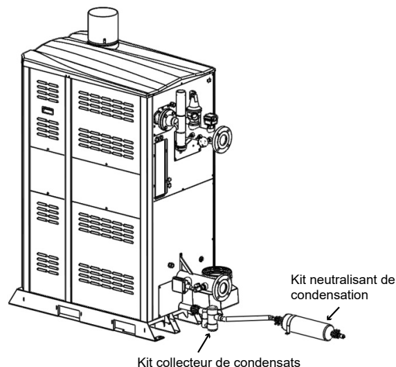
Figure 82. Guide visuel pour la tuyauterie de condensat
