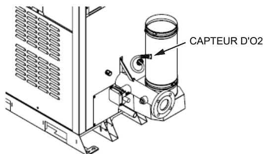
Figure 95. O2 Emplacement du capteur
