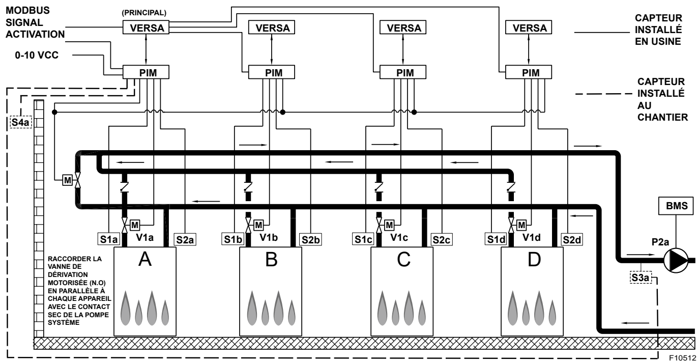
Figure 33. Cascade de chaudières (jusqu'à 8 appareils) avec vanne de dérivation motorisée
