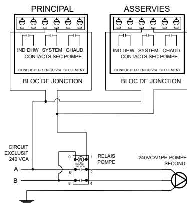
Figure 55. Pompes système en cascade (240 VCA illustré)
