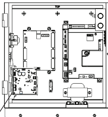
Figure 94. Emplacement de la carte HO2T à l'intérieur de la J-Box
