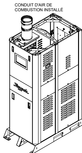
Figure 18. Installation d'un conduit d'air de combustion
