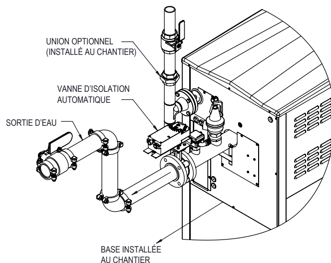
Figure 21. Installation de la vanne d'isolation motorisée
