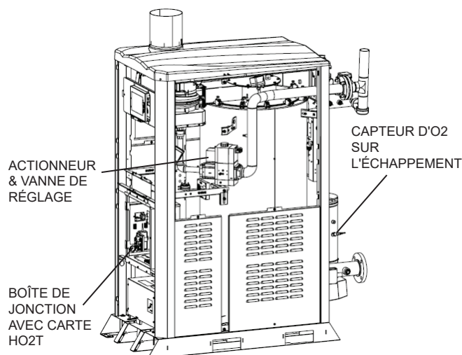
Figure 93. Composants du système de surveillance O2
