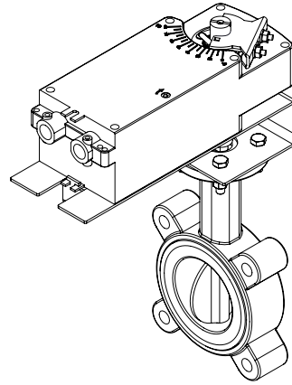
Figure 48. Vanne d'isolation motorisée
