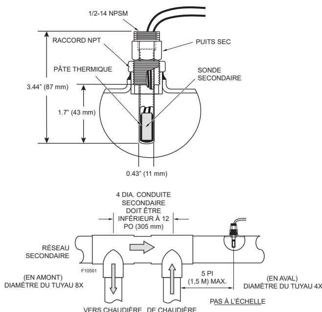
Figure 23. Installation de la sonde système, primaire/secondaire
