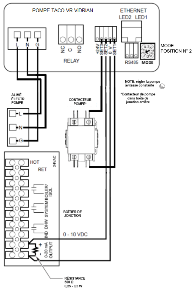
Figure 54. Schéma de câblage, pompe VS
