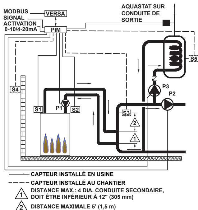
Figure 27. Mode 1 - Cascade de chaudières recommandée (jusqu'à 8 appareils) - boucles prim./sec.
