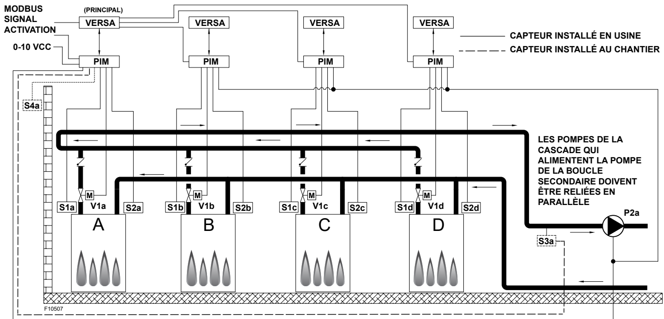
Figure 32. Mode 1 - Cascade de chaudières recommandée (jusqu'à 8 appareils) - boucle primaire
