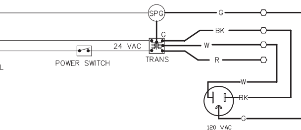
Figure 35. Câblage modèle P-106
