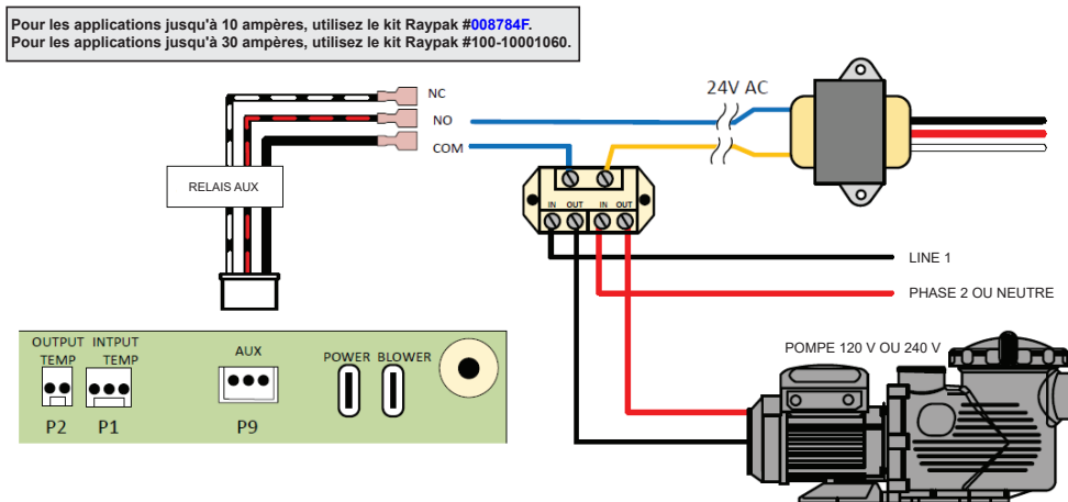
Figure 134. Application haute puissance avec relais SPDT (non fourni)
