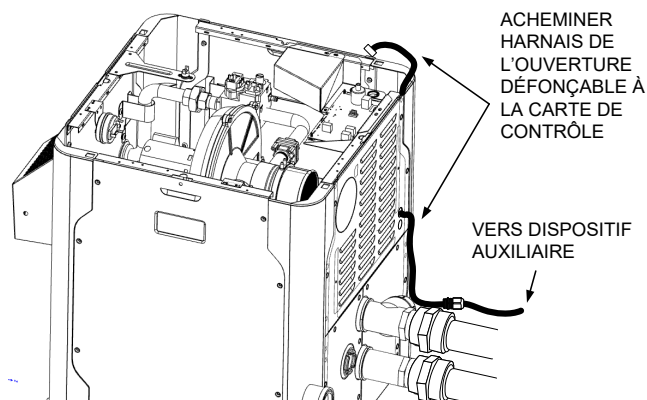
Figure 131. Acheminement du harnais de communication
