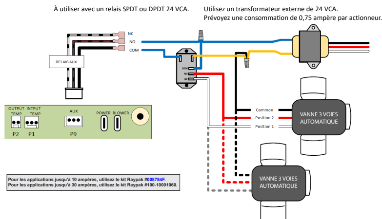
Figure 133. Vanne à 3 voies
