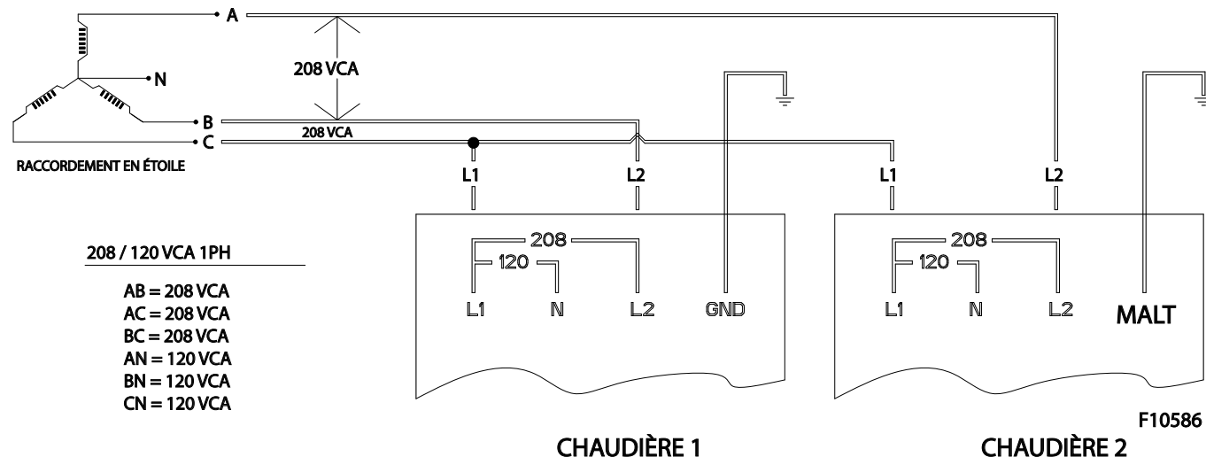
Figure 34. Raccordement électrique en étoile 120/208 VCA
