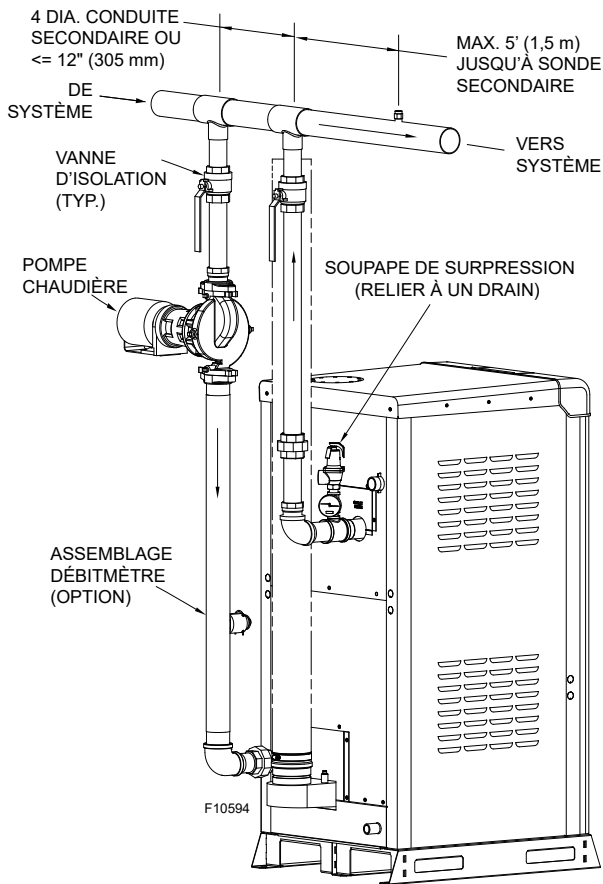
Figure 17. Boucles primaire/secondaire hydroniques
