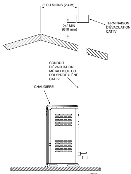
Figure 41. Acier inoxydable et polypropylène - Ventilation verticale
