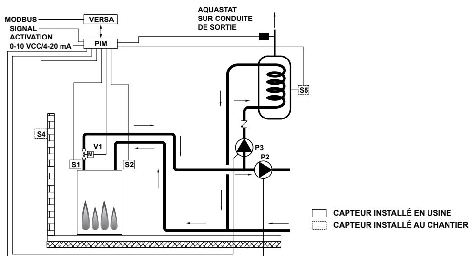
Figure 29. Mode 2 - Chaudière unique avec chauffe-eau indirect - boucle primaire
