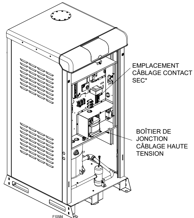
Figure 32. Emplacement de la boîte de jonction
