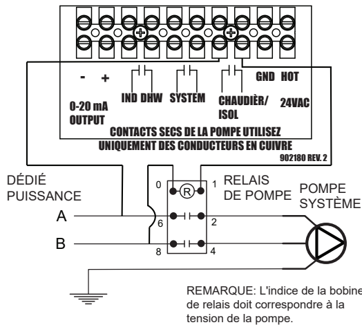
Figure 38. Schéma de câblage de la chaudière (l'indice de bobine de relais doit correspondre à la tension nominale de la pompe)
