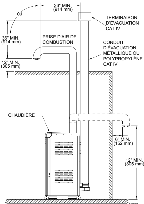
Figure 42. Acier inoxydable et polypropylène - Ventilation directe verticale
