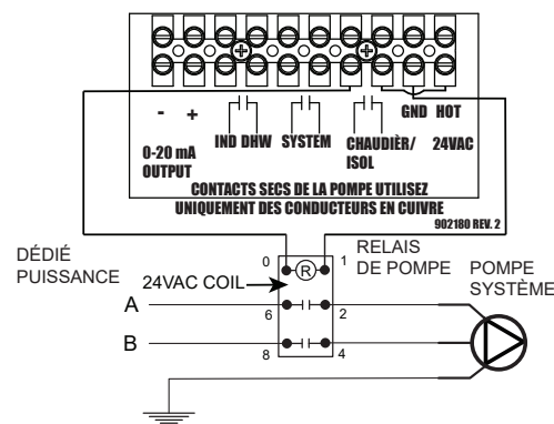
Figure 37. Schéma de câblage de la pompe de chaudière (relais de bobine 24VAC)
