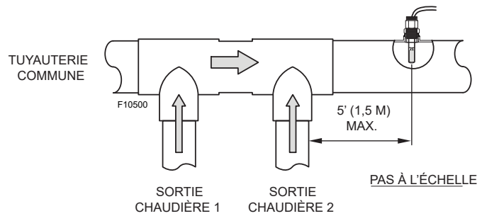
Figure 16. Installation de la sonde système, primaire système en cascade
