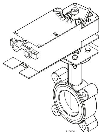
Figure 68. Vanne d'isolation automatique
