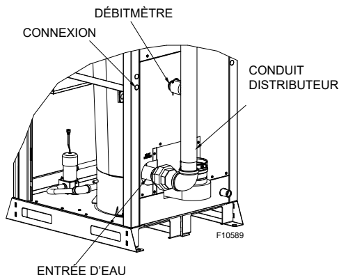
Figure 62. Débitmètre
