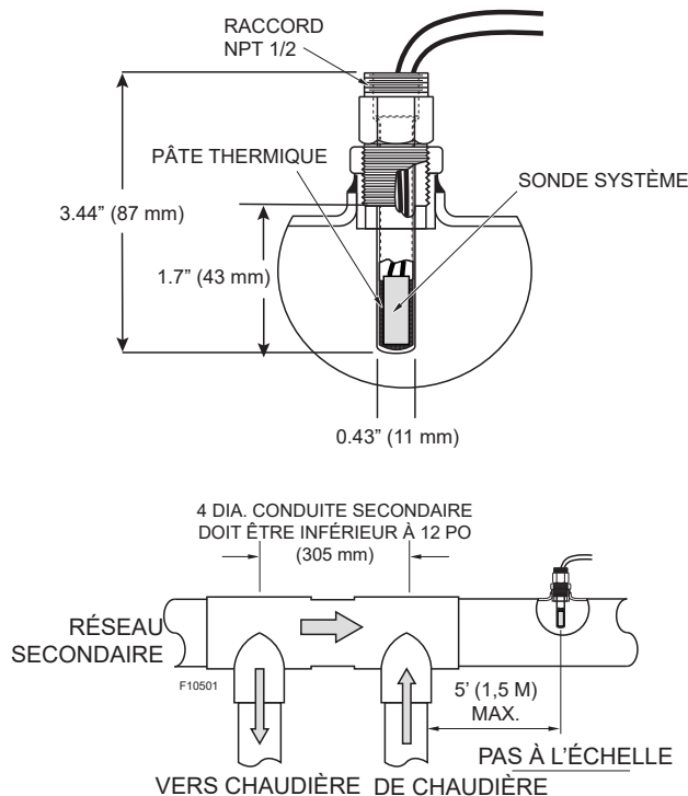
Figure 15. Installation de la sonde système, primaire/secondaire
