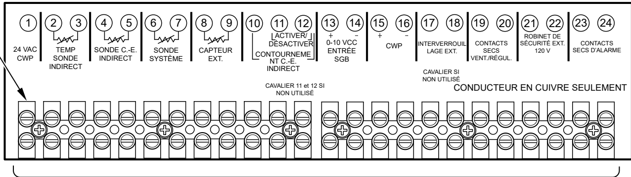
Figure 35. Câblage basse tension au chantier
