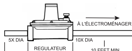
Figure 31. Distances de régulateur de gaz
