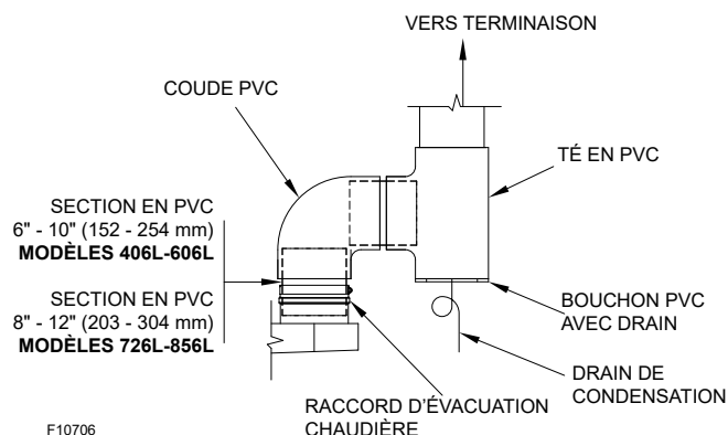
Figure 49. Détails de l'assemblage en PVC - Installation au chantier
