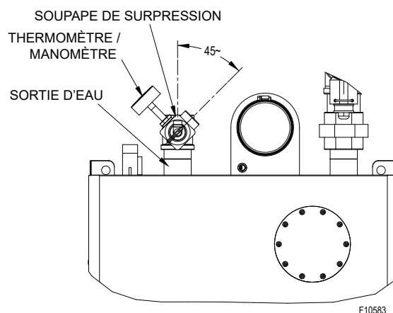
Figure 14. Orientation recommandée de la soupape
