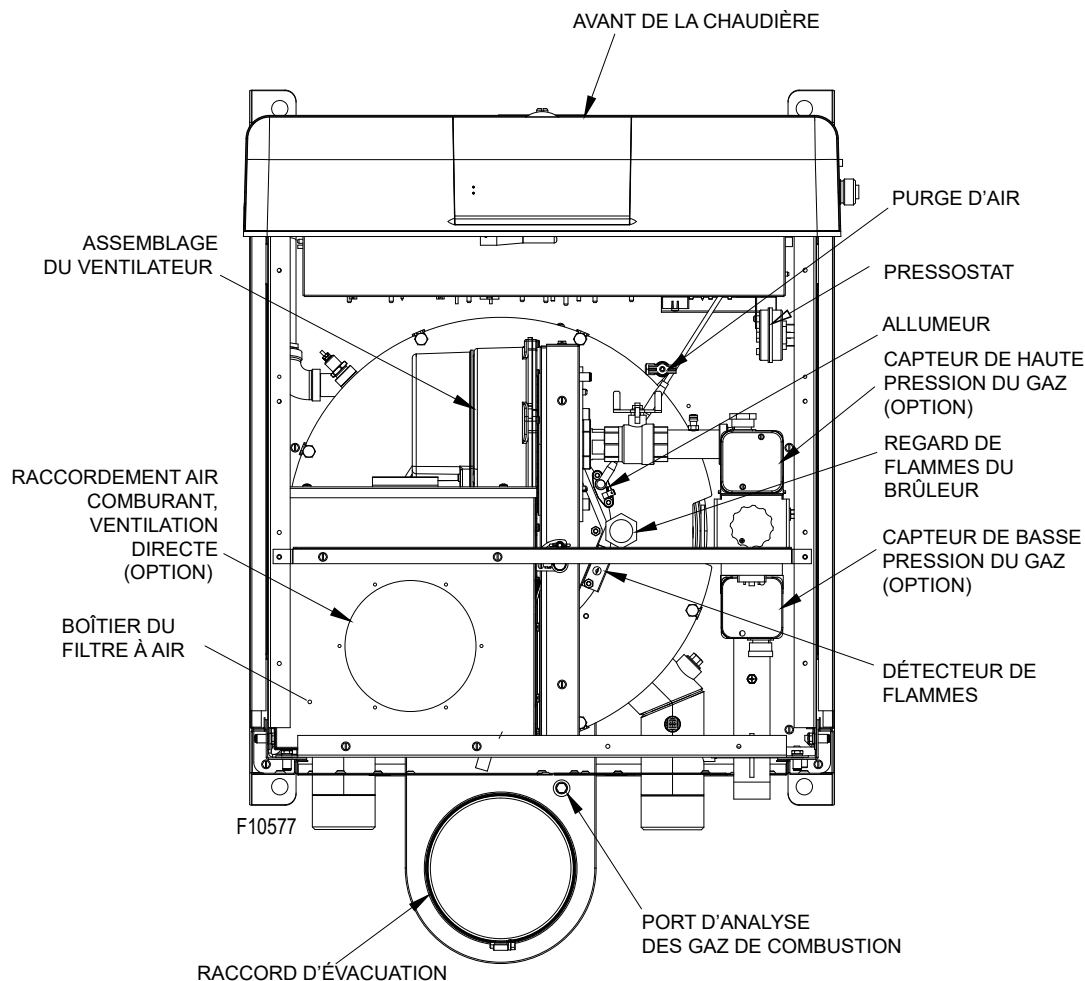
Figure 5. Position des pièces – Vue du dessus
