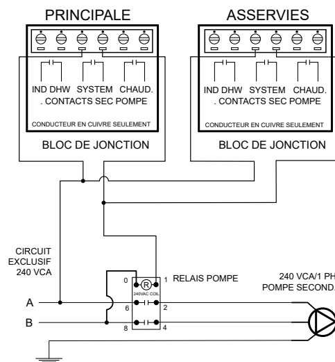
Figure 40. Pompes système en cascade XVersL (240 VCA illustré)
