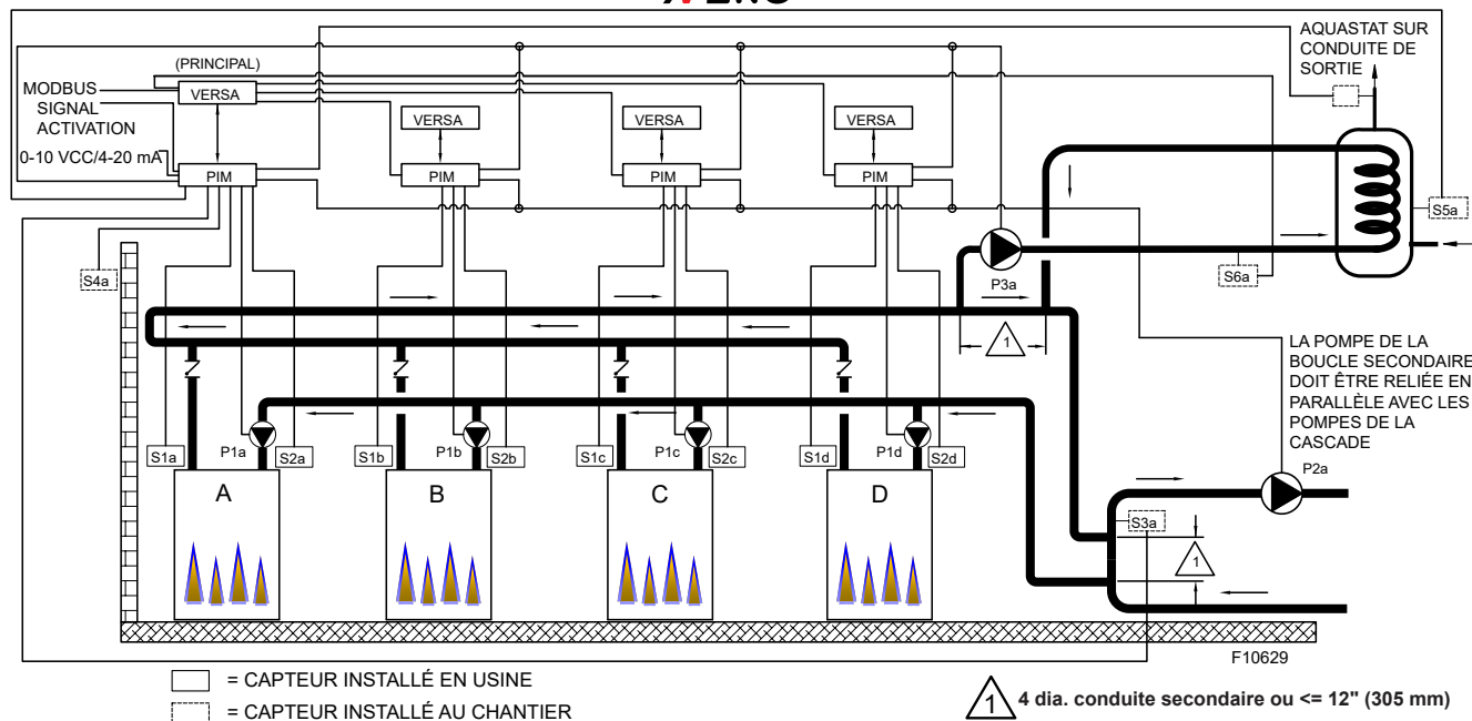
Figure 23. Mode 3 - Chaudières en cascade avec chauffe-eau indirect, boucle primaire/secondaire
