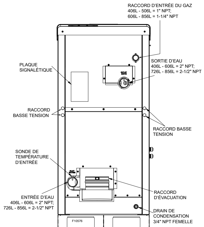
Figure 4. Position des pièces – Vue arrière
