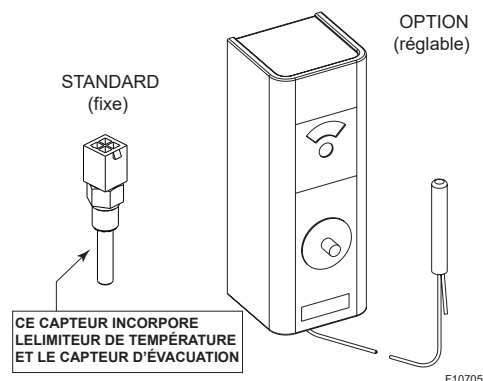
Figure 69. Limiteur de température à réarmement manuel
