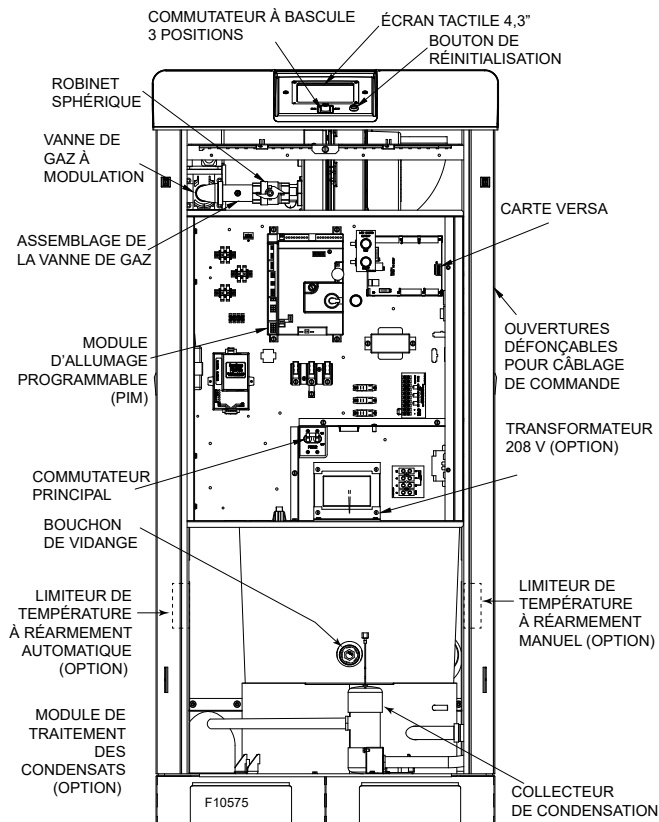
Figure 3. Position des pièces – Vue avant
