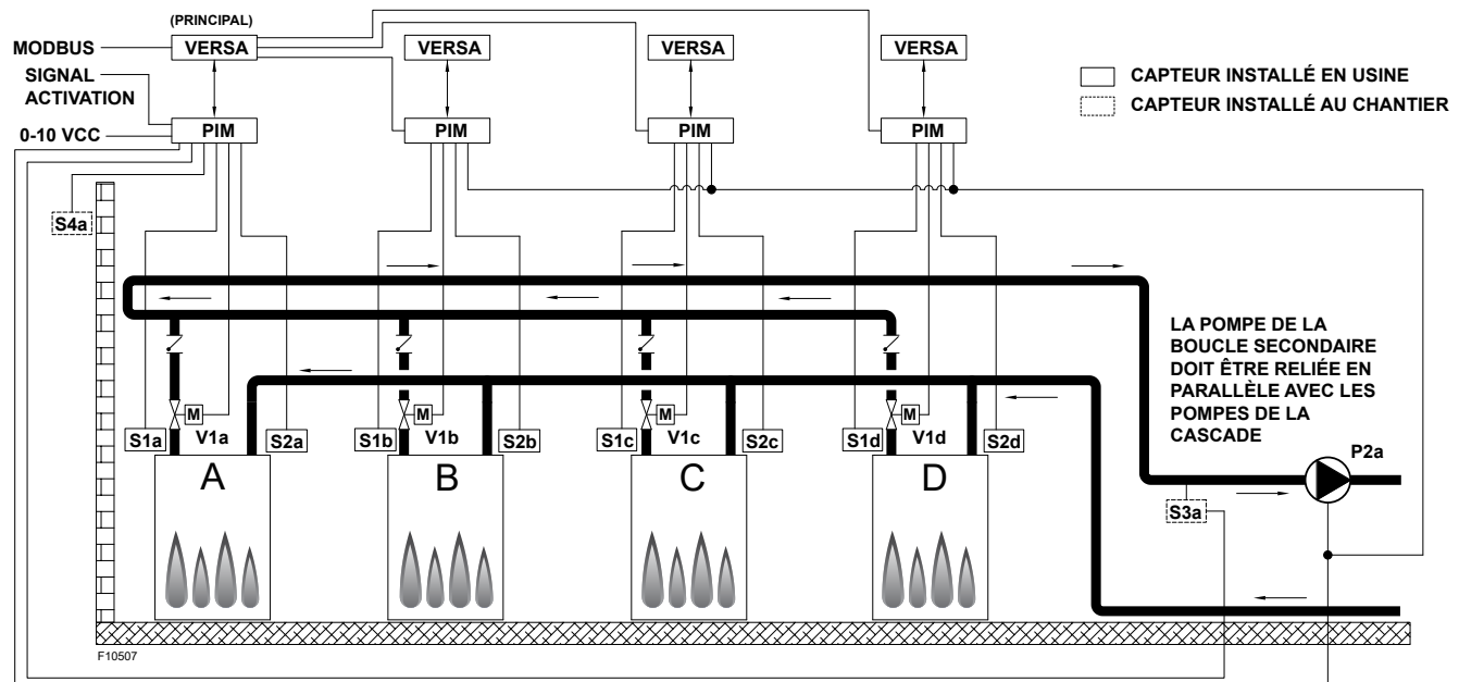
Figure 26. Mode 1 - Chaudières en cascade avec boucles primaire
