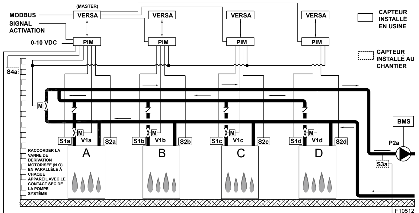
Figure 27. Cascade de chaudières avec vanne de dérivation motorisée
