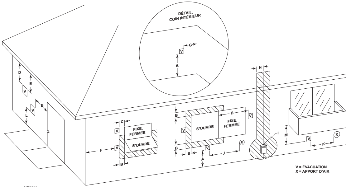
Figure 12. Dégagements minimum aux matières combustibles, terminaisons d'apport d'air et d'évacuation – Installation intérieure ou extérieure
