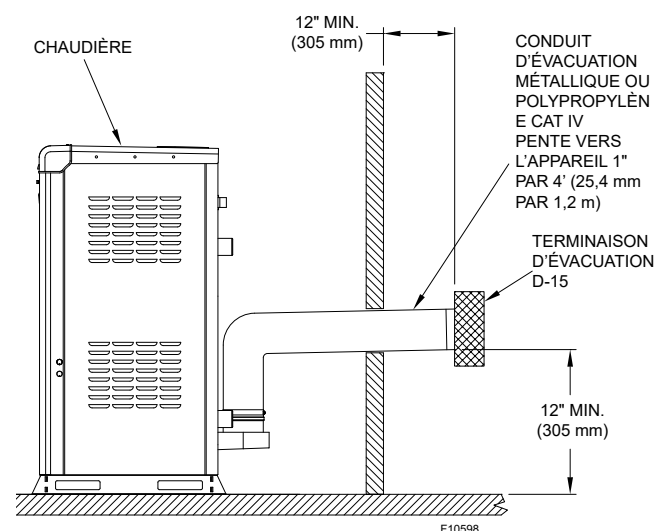
Figure 43. Acier inoxydable et polypropylène - Ventilation directe murale à l'horizontale
