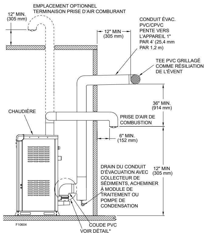
Figure 49. Détails de l'assemblage en PVC - Installation au chantier
