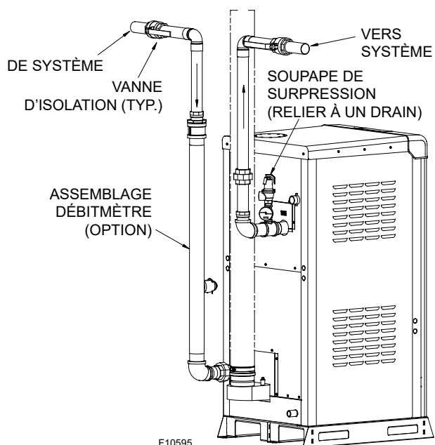
Figure 24. Tuyauterie primaire hydronique
