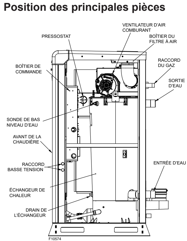
Figure 2. Position des pièces – Vue de côté
