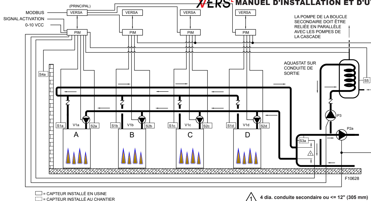
Figure 21. Mode 2 - Chaudières en cascade avec chauffe-eau indirect sur la boucle secondaire
