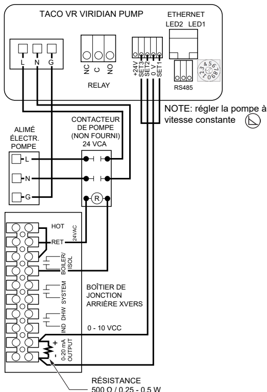
Figure 39. Schéma de câblage de la pompe à vitesse variable
