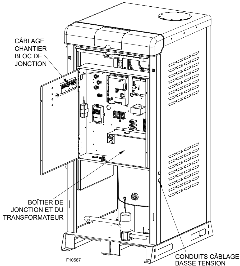
Figure 36. Boîtier de jonction basse tension
