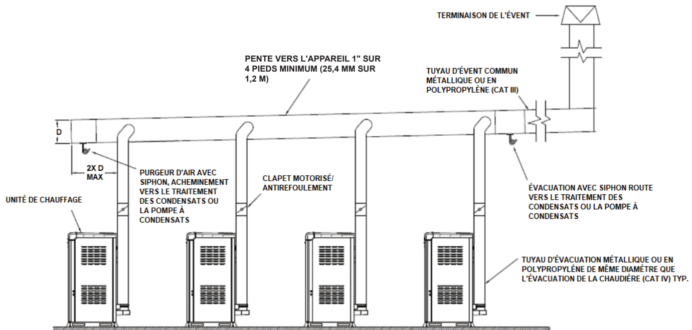
Figure 53. Évent commun à pression positive typique
