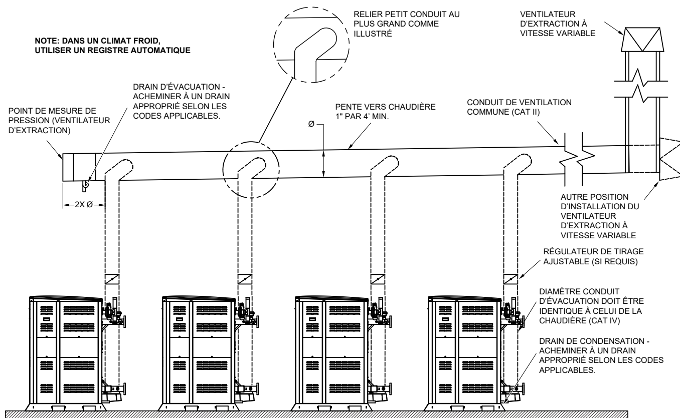
Figure 52. Évent commun à pression négative typique
