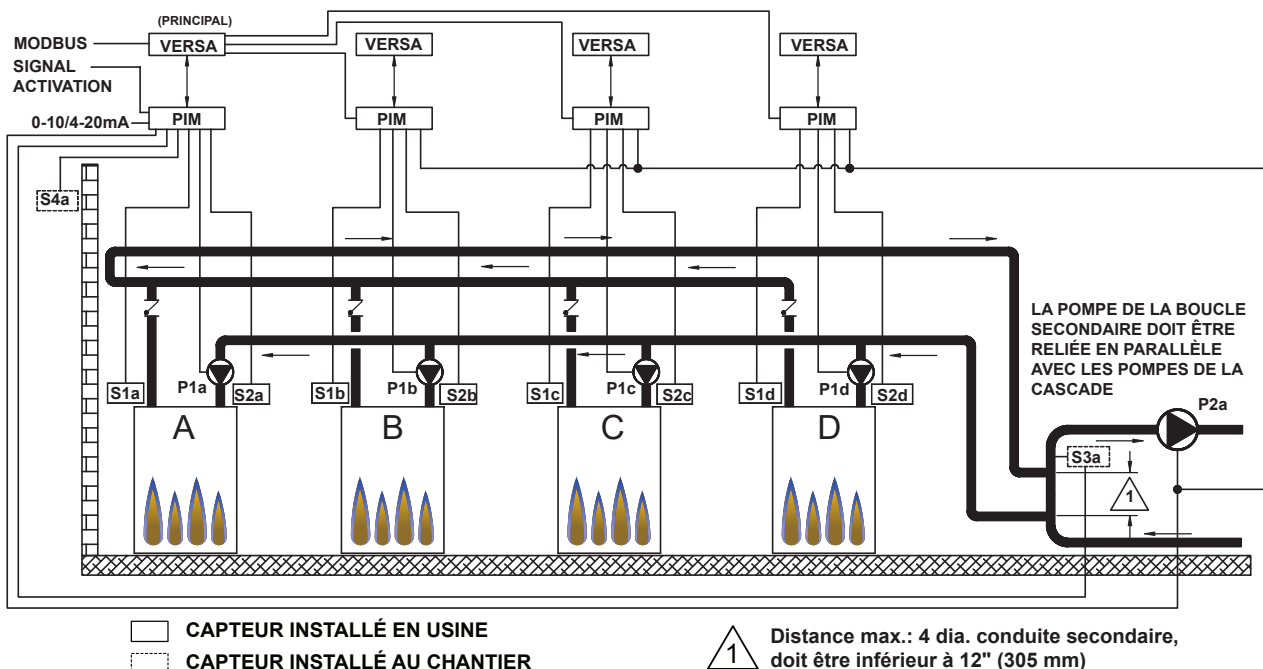
Figure 19. Mode 1 - Chaudières en cascade avec boucles primaire/secondaire
