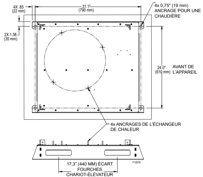
Figure 8. Ancrage pour un appareil
