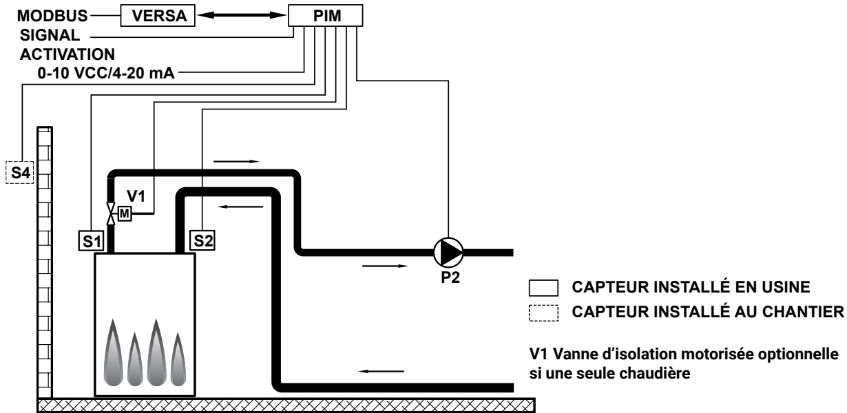
Figure 25. Mode 1 - Chaudière unique avec boucle primaire
