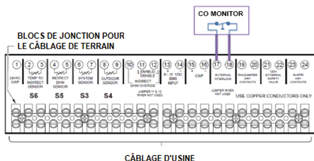
Figure 54. Câblage de terrain basse tension (moniteur CO)
