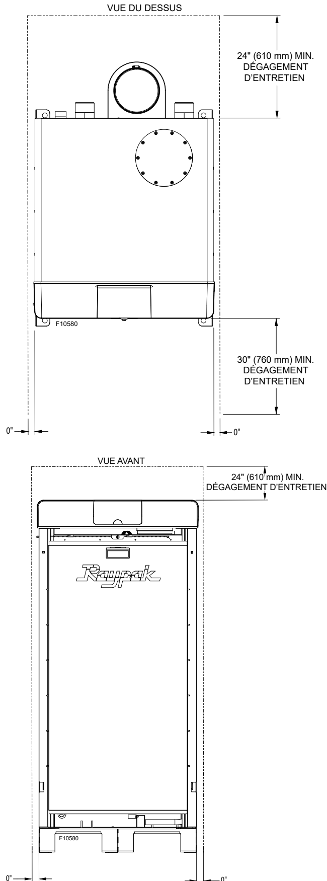
Figure 10. Dégagements minimum aux matières combustibles – Installation intérieure ou extérieure
