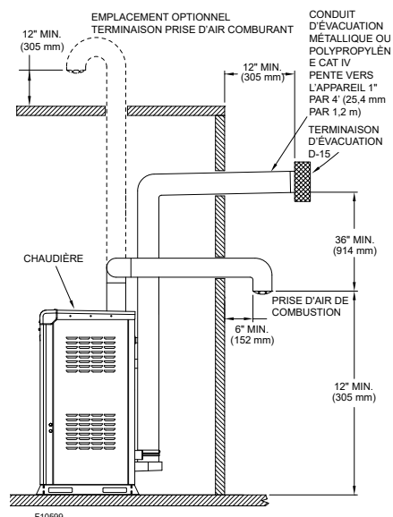
Figure 44. Acier inoxydable et polypropylène - Ventilation directe à l'horizontale
