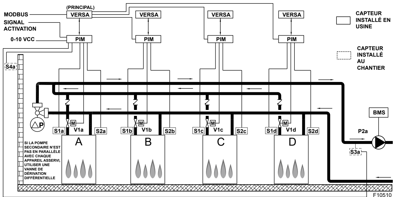
Figure 28. Cascade de chaudières avec vanne de dérivation à pression différentielle - boucle primaire
