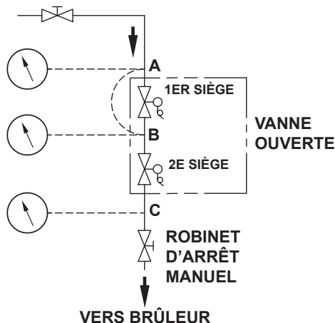
Figure 46. Essai d'étanchéité
