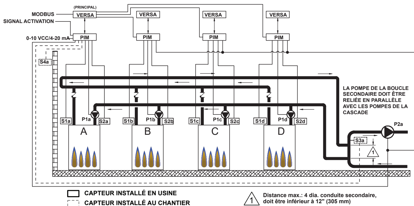
Figure 14. MODE 1 - Chaudières en cascade avec boucles primaire/secondaire
