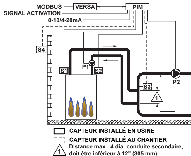
Figure 13. Mode 1 - Chaudière unique avec boucles primaire/secondaire
