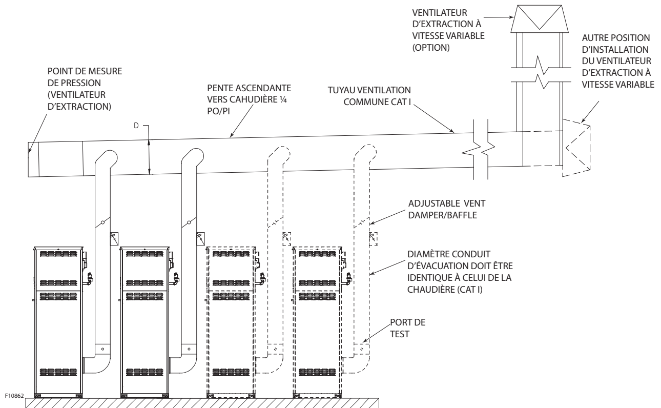
Figure 29. Ventilation commune typique
