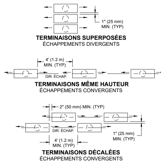
Figure 27. Disposition des terminaisons d'évacuation
