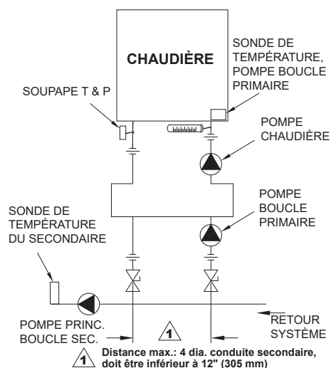
Figure 10. Fonctionnement à l'eau froide
