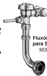
Fluxómetro para Mingitorio para Spud Superior de 1 1/4" MODELO 180 Fluxómetro para Mingitorio para Spud Superior de 3/4" MODELO 186
