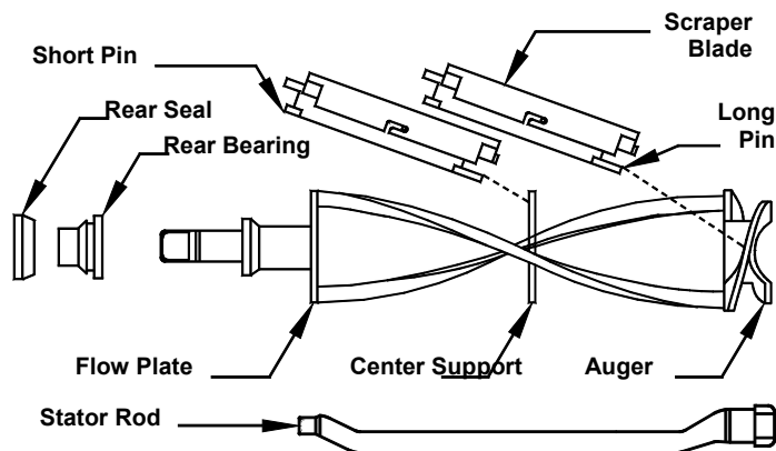
Fig. 10(b) 521 & 522 Dasher Assembly
