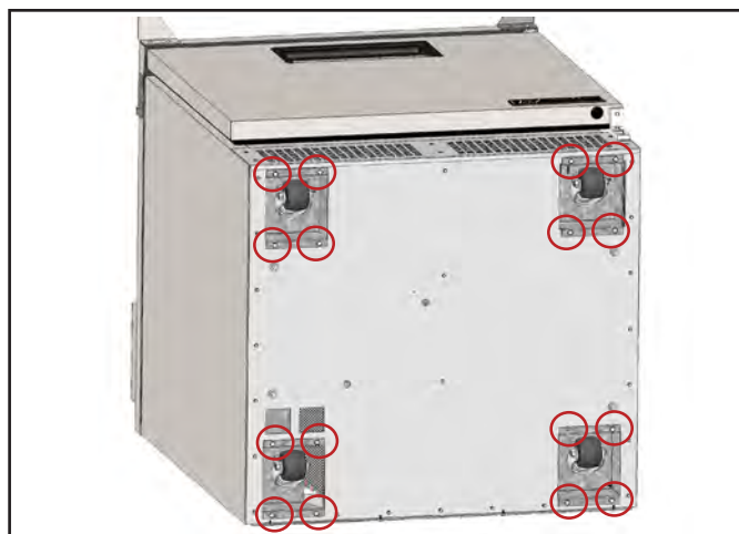
Fig. 11. Localice la carcasa de la rueda. Retire los cuatro tornillos que aseguran la carcasa.
