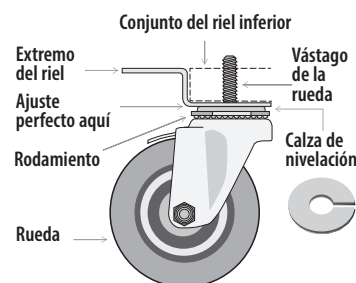
Fig. 7. Representación esquemática de una rueda.
