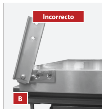
Fig. 8. Las imágenes muestran la parte delantera de la puerta mirando hacia arriba.
