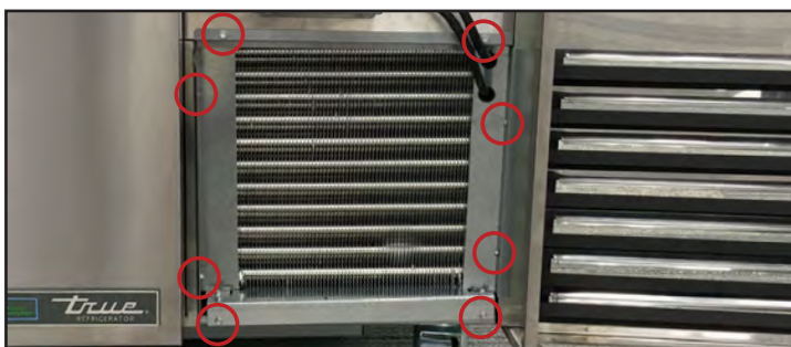
Fig. 5. Retire los soportes del condensador, si los hay.
