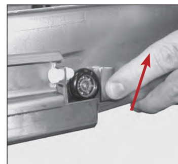
Fig. 4. Levante y retire el cajón.
