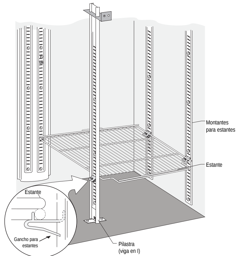
Fig. 3. Tal vez deba apretar o girar la parte inferior del gancho para estantes para instalarlo.
