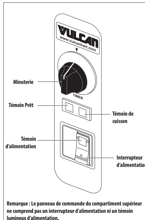
Figure 2 Commandes de l'armoire
